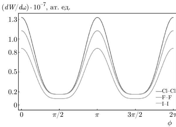
Рис. 4. (В цвете онлайн) Зависимости спектральной плотности излучения молекулярных анионов хлора, фтора и йода от угла падения \phi (угол между \mathbf{E}_0 и \mathbf{R} ) фотона
