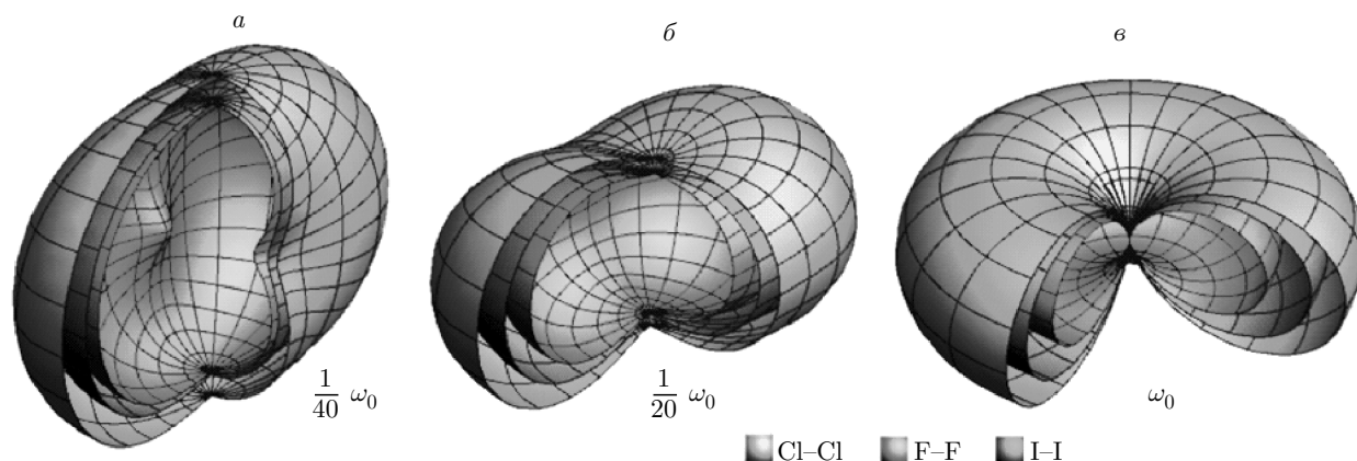
Рис. 5. (В цвете онлайн) Эволюция диаграммы направленности рассеяния ультракороткого импульса электромагнитного поля анионов (хлора, фтора, йода) на второй гармонике в зависимости от несущей частоты падающего УКИ при \omega_0 \approx 660 ат.ед. (ось z по направлению падающего импульса)
