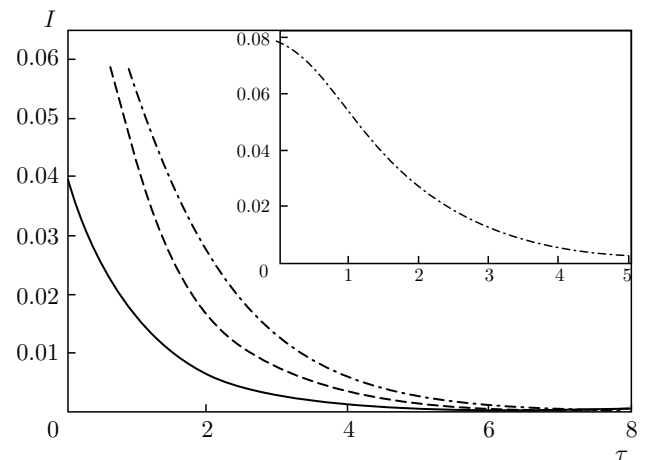
Рис. 5. Интенсивность низкочастотного импульса полувозбужденного ансамбля с числом частиц, большим критического. Параметры штарковского взаимодействия рабочих уровней различные \eta_- = \pi/4 . Сплошная кривая — \eta_+ = \pi/4 + 1.3 , штриховая кривая — \eta_+ = \pi/4 + 1.45 , штрихпунктирная кривая — \eta_+ = \pi/4 + 1.6 . Эта кривая отдельно представлена на вставке
