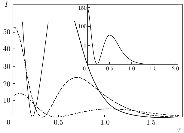
Рис. 4. Интенсивность низкочастотного импульса полувозбужденного ансамбля с числом частиц, меньшим критического. Параметры штарковского взаимодействия рабочих уровней разные \eta_- = \pi/4 . Сплошная кривая — \eta_+ = \pi/4 + 0.4 (эта кривая отдельно представлена на вставке), штриховая кривая — \eta_+ = \pi/4 + 0.5 , штрихпунктирная кривая — \eta_+ = \pi/4 + 0.6
