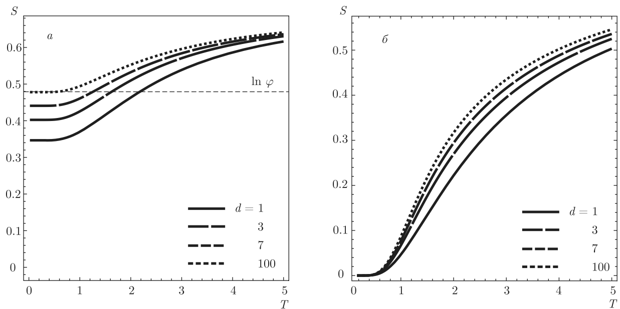
Рис. 5. Температурные зависимости энтропий в точках фрустраций антиферро-ферромагнитной модели Изинга ( J_d = -1 , J = 1 ) для различных значений декорирования цепочки: a — в магнитном поле H = 2 , б — в магнитном поле H = 4
