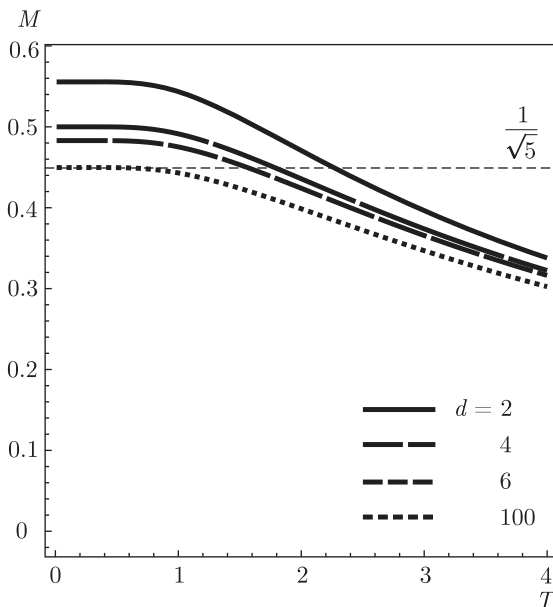
Рис. 7. Температурные зависимости намагниченности при d = 2, 4, 6, 100 ( J_d = -1 , J = 1 ) при H = 2 . Видно, что при стремлении d к бесконечности, значение нуль-температурной намагниченности становится равно 1/\sqrt{5}
