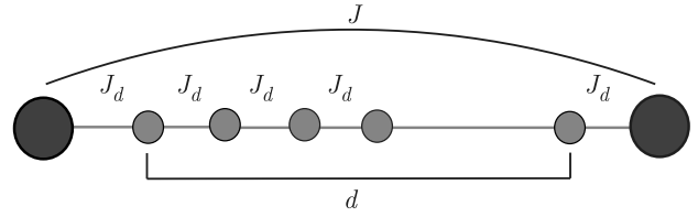
Рис. 1. Декорированная цепочка с обменным взаимодействием ближайших соседей J_d и обменным взаимодействием J
