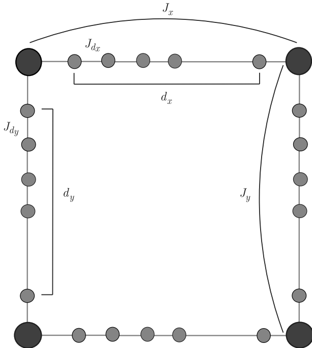
Рис. 12. Декорированная квадратная решетка с обменными взаимодействиями ближайших соседей J_{dx} и J_{dy} соответственно по горизонтальному и вертикальному направлению, а также с обменными взаимодействиями J_x по направлению x и с обменными взаимодействиями J_y по направлению y
