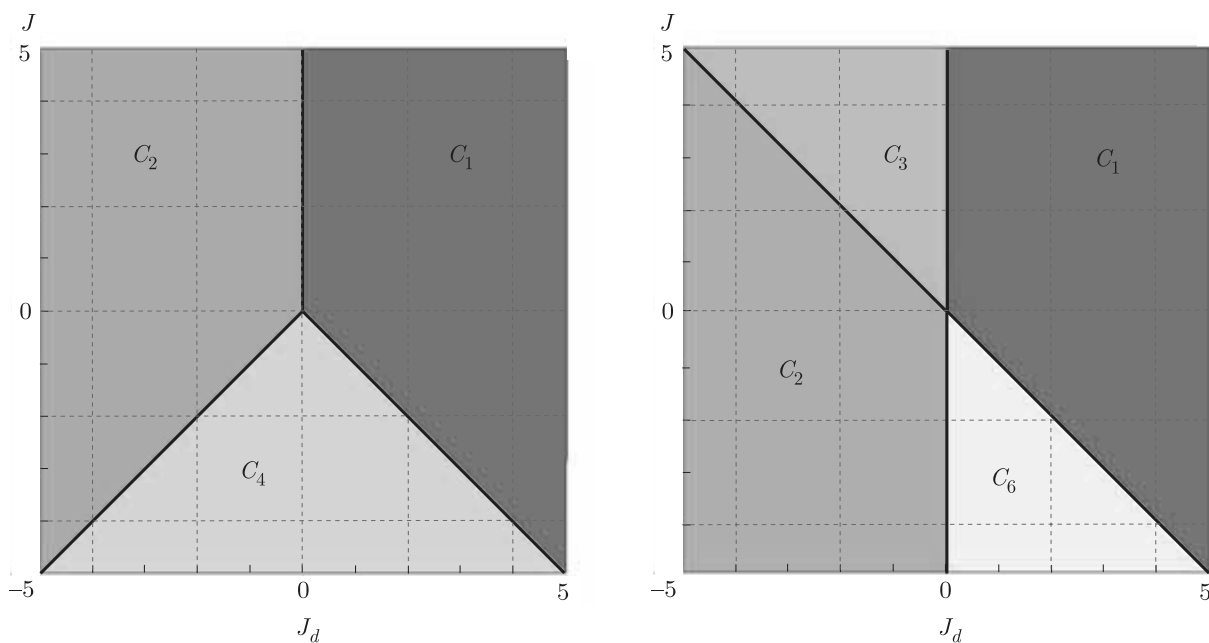
Рис. 11. Фазовые диаграммы основного состояния системы декорированной изинговской цепочки в отсутствие магнитного поля: а — при d = 1 , б — при d = 2
