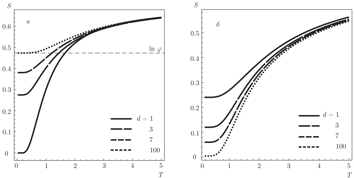
Рис. 2. Температурные зависимости энтропий в точках фрустраций антиферромагнитной модели Изинга ( J_d = -1 , J = -1 ) для различных значений декорирования цепочки: a — в магнитном поле H = 2 ; б — в магнитном поле H = 4
