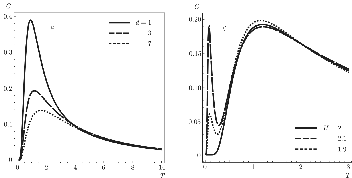
Рис. 3. Температурные зависимости теплоемкостей при различных значениях декорирования d : a — теплоемкость всегда равна нулю при стремлении температуры к нулю или к бесконечности ( H = 2 для всех кривых), б — расщепление теплоемкости на два пика вблизи фрустрации
