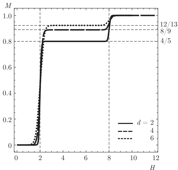
Рис. 13. Намагниченность антиферромагнитной модели Изинга двукратно-, четырехкратно- и шестикратно-декорированной квадратной решетки ( J_{dx} = -1 , J_{dy} = -1 , J_x = -1 , J_y = -1 ) при T = 0.005
