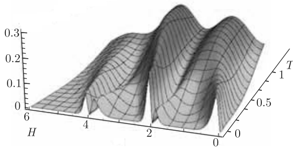
Рис. 8. Теплоемкость трижды декорированной ( d = 3 ) антиферромагнитной модели Изинга ( J_d = -1 , J = -1 ) как функция температуры и магнитного поля
