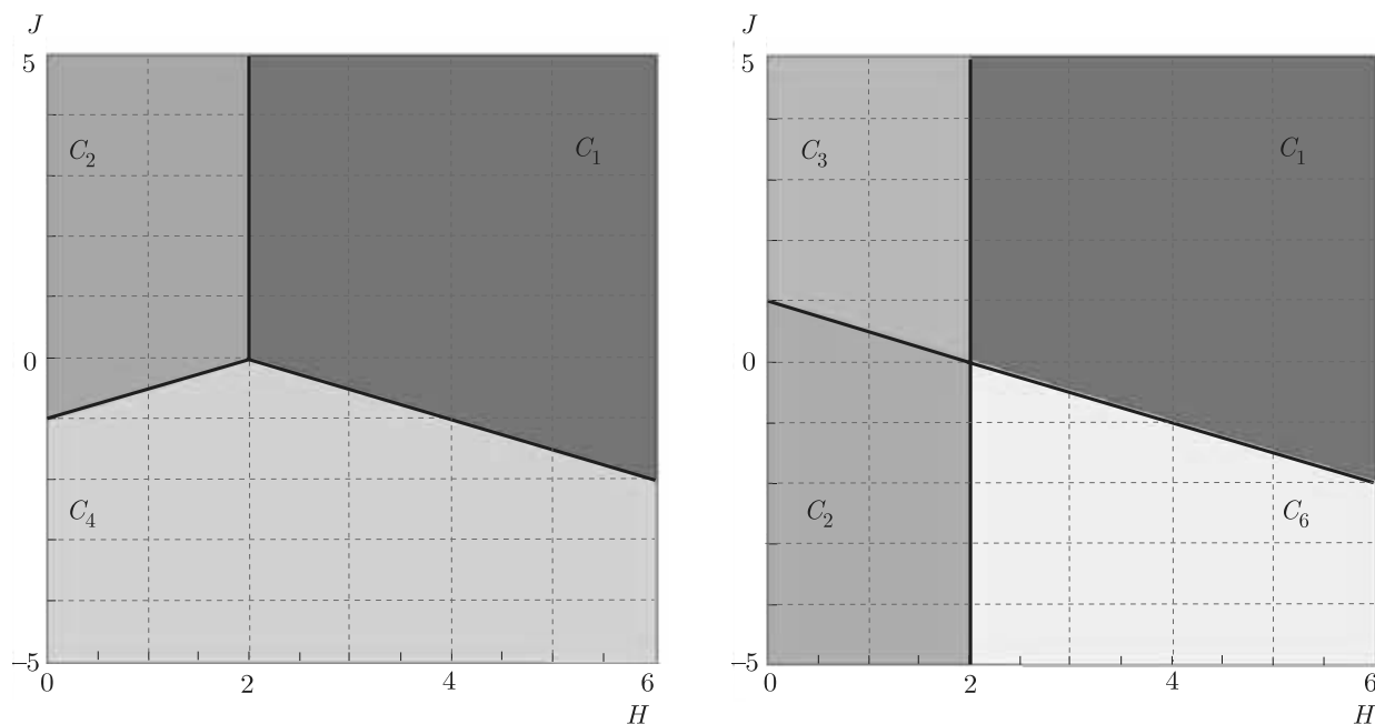
Рис. 10. Фазовые диаграммы основного состояния системы декорированной изинговской цепочки в магнитном поле с учетом обменного взаимодействия между ближайшими соседями J_d = -1 : а — при d = 1 , б — при d = 2
