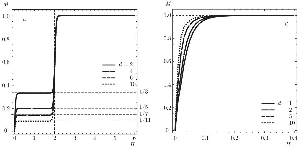
Рис. 6. Намагниченность антиферро-ферромагнитной модели Изинга ( J_d = -1 , J = 1 ) при температуре T = 0.06 для четных значений декорирования цепочки (а), ферро-антиферромагнитной модели Изинга ( J_d = 1 , J = -1 ) при температуре T = 0.06 для различных значений декорирования цепочки (б)
