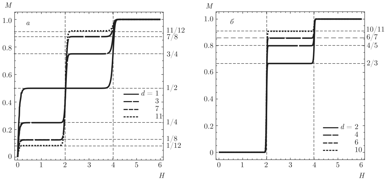
Рис. 4. Намагниченность антиферромагнитной модели Изинга ( J_d = -1 , J = -1 ) для различных значений декорирования цепочки: a — нечетные значения d при температуре T = 0.06 , б — четные значения d при температуре T = 0.02
