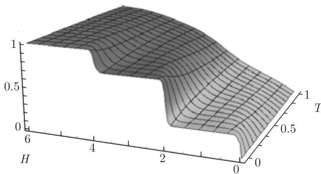
Рис. 9. Намагниченность трижды декорированной ( d = 3 ) антиферромагнитной модели Изинга ( J_d = -1 , J = -1 ) как функция температуры и магнитного поля
