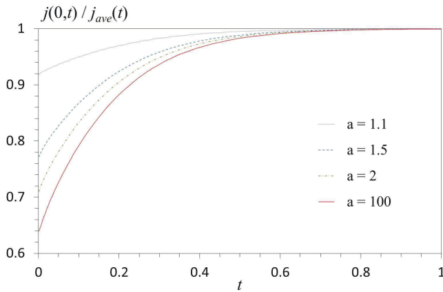
Рис. 7. Зависимость от времени отношения плотности тока при x = 0 к среднему значению тока в фольге j_{ave}(t) для различных расстояний между фольгами
