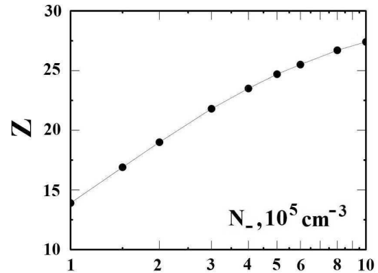
Рис. 1. Заряд Z растущих микрокапель в кучевом облаке в зависимости от плотности N_+ положительных ионов в соответствии с уравнением (7)
