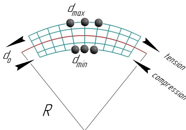
Рис. 4. Возникновение деформаций растяжения–сжатия при цилиндрическом изгибе алмазной пластины с ориентацией поверхности (110)
