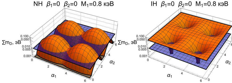
Рис. 2. Поверхности, иллюстрирующие масштаб величины \sum_{\alpha} (m_D)_{\alpha 1} в зависимости от углов \alpha_1 и \alpha_2 , параметризующих вещественную ортогональную матрицу \Omega для случаев прямой иерархии масс активных нейтрино (левая панель) и обратной (правая панель). Синяя плоскость — верхняя граница (m_D)_{\chi\text{-ray}} (см. (25)), полученная из ограничений на время жизни \tau_{N_1} > 10^{25} с [24] и взятая при массе стерильного нейтрино темной материи M_1 = 0.8 кэВ
