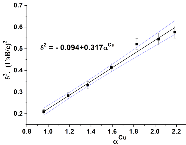
Рис. 5. Показатель экспоненты \delta^2 как функция \alpha^{\text{Cu}} . Корridor ошибок соответствует одному стандартному отклонению
