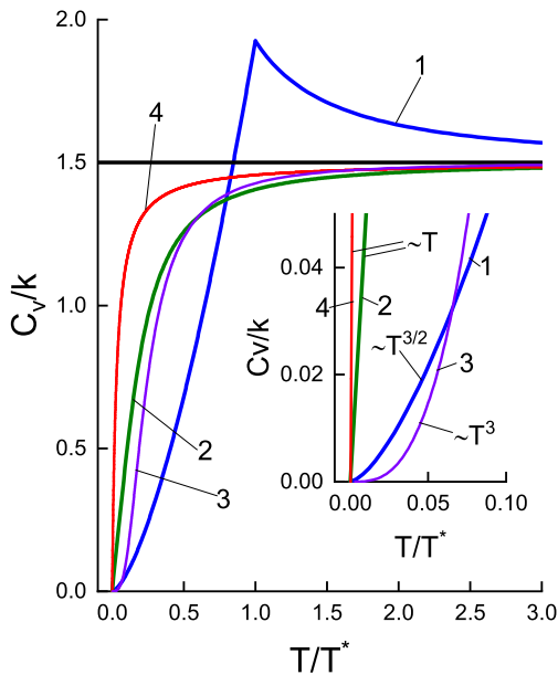
Рис. 6. Нормированные теплоемкости модельных систем (1 — C_v идеального бозе-газа, T^* = T_c — температура фазового перехода, 2 — C_v идеального ферми-газа, T^* = T_{Fermi} , 3 — C_v of Debye solid, T^* = T_\theta — температура Дебая, 4 — C_v квантовой системы твердых сфер,
