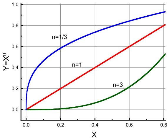
Рис. 5. Функции вида Y = X^n в окрестности x=0
