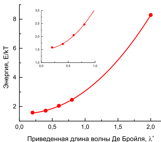
Рис. 1. Зависимость безразмерной энергии E/kT жидкости квантовых твердых сфер от приведенной длины волны де Бройля \lambda^* = h/(2\pi m k T \sigma^2)^{1/2} , кружки — результаты расчетов [7], линия — аппроксимация
