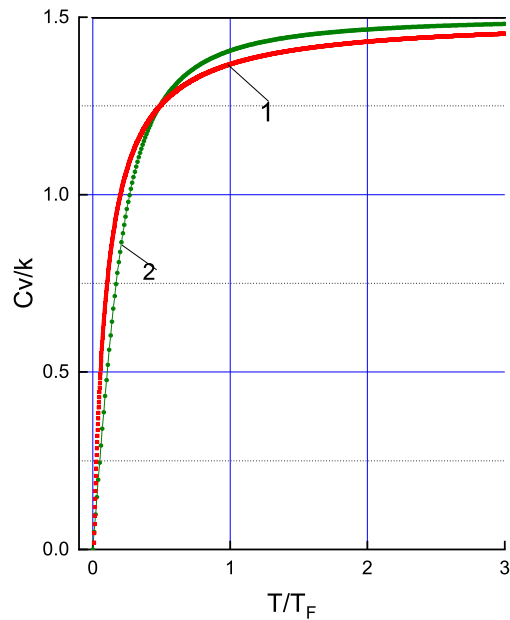
Рис. 7. Приведенная теплоемкость квантовой системы твердых сфер (1) по сравнению с теплоемкостью идеального ферми-газа (2)
