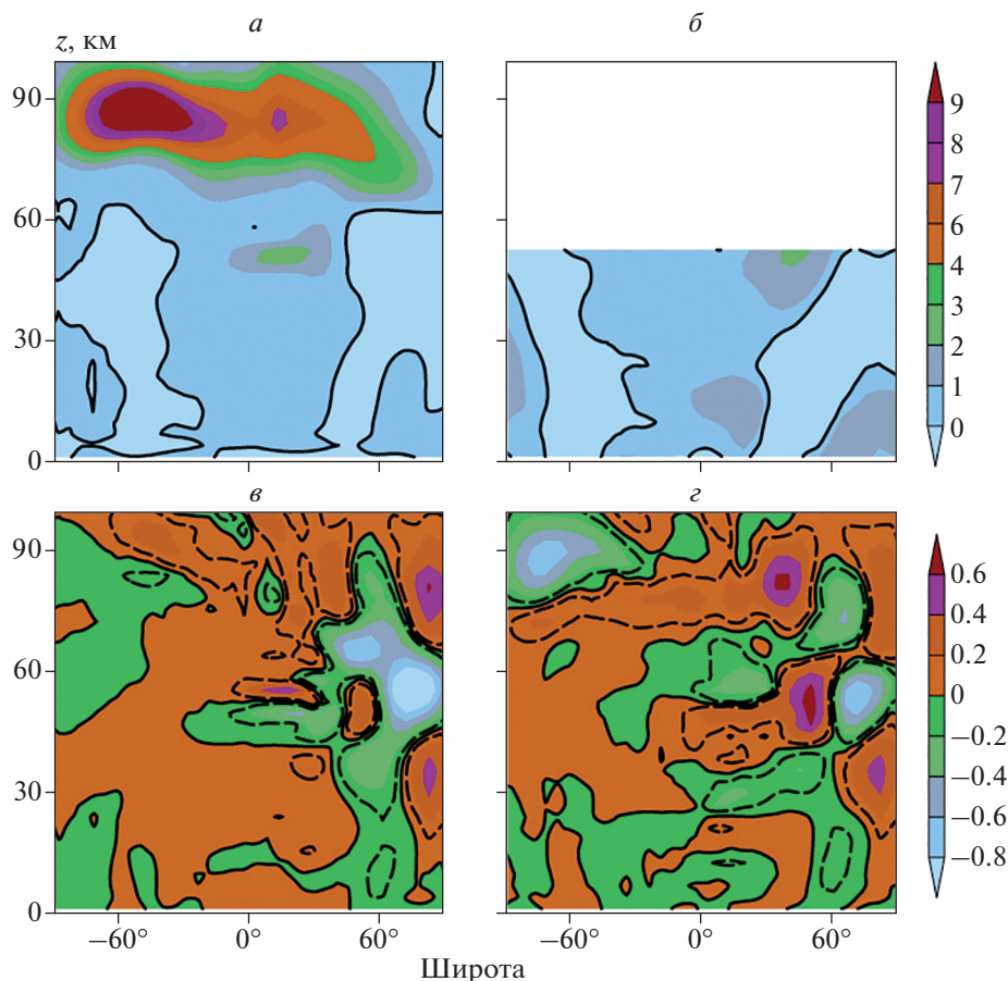
Рис. 1. Средние широтно-высотные распределения меридиональной скорости (в м/с) для января, рассчитанные по модели МСВА без учета параметризации ОГВ (а) и полученные из данных реанализа JRA-55 (б). Приращения меридиональной скорости (в м/с) за счет воздействия ОГВ (в) и за счет перехода от восточной к западной фазе КДК (з). Сплошные линии показывают нулевые значения, штриховые — границы областей с 95%-ной значимостью ненулевых приращений.
