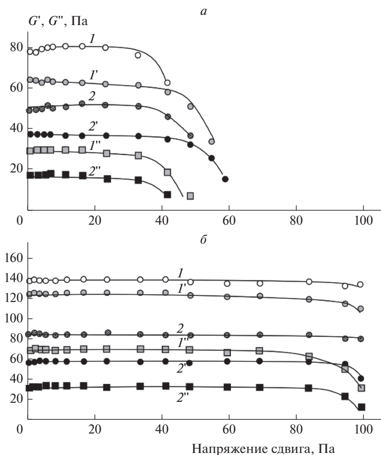
Рис. 4. Зависимость модулей накоплений ( G' , G'' ) и потерь ( 2 , 2' , 2'' ) от напряжения сдвига для гелей на основе ПЭК-0.5 (а) и ПЭК-1 (б). Частота осциллирующего напряжения – 1 Гц; амплитуда напряжения – 1 Па; 1, 2 – буферный раствор (рН = 6.86); 1', 2' – \text{H}_2\text{O} ; 1'', 2'' – 0.25 М раствор NaCl.
