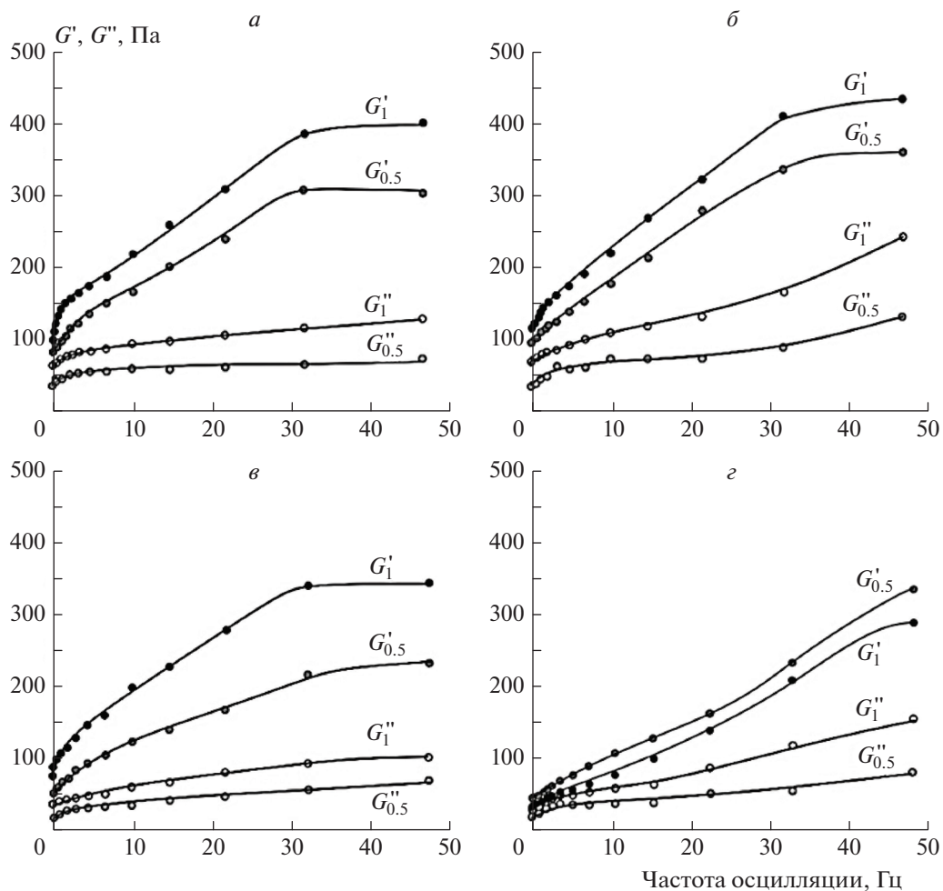
Рис. 5. Зависимость модулей накоплений и потерь от частоты осцилляции для гелей на основе ПЭК-0.5 и ПЭК-1 в различных средах: a – бидистиллированная вода; б – фосфатный буферный раствор; в – 0.05 М раствор NaCl; г – 0.25 М раствор NaCl.
