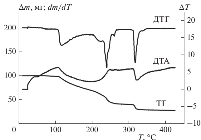
Рис. 2. Дериватограмма порошковой смеси ГНН + 0.1 ГМТА в потоке азота; m = 100 мг, V = 20^\circ/\text{мин} .
