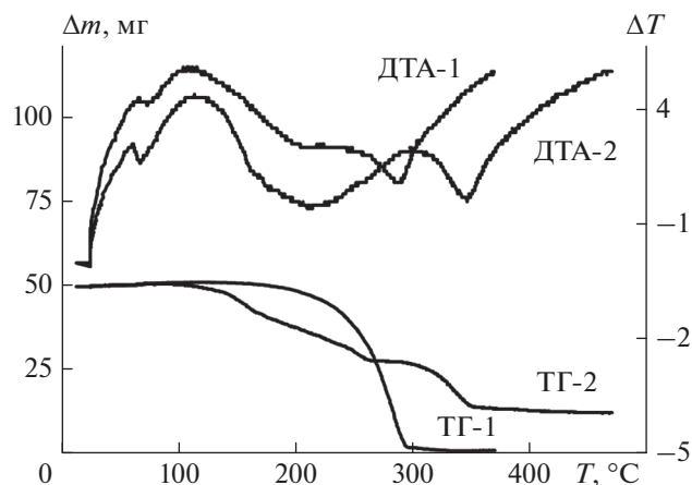
Рис. 1. ДТА/ТГ-кривые разложения ГМТА (1) и ГНН (2); V = 20^\circ\text{C}/\text{мин} , m = 50 мг.
