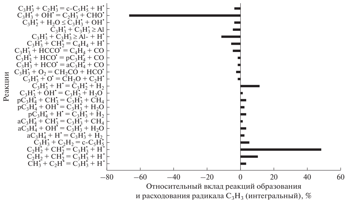
Рис. 13. Основные реакции образования и расхода радикалов C_3H_3 для смеси 0.5CH_4 + 0.3O_2 + 0.2CO_2 ( \phi = 3.33 ), T_{50} = 1800 К и P_{50} = 1 бар.
