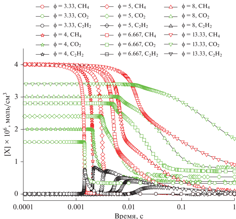
Рис. 1. Расчет изменения концентрации CH 4 , CO 2 и C 2 H 2 для различных значений \phi при T_{50} = 1500 К и P_{50} = 1 бар.
