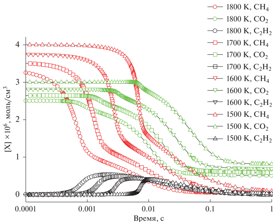
Рис. 7. Расчет изменения концентрации \text{CH}_4 , \text{CO}_2 , и \text{C}_2\text{H}_2 для смеси 0.5\text{CH}_4 + 0.125\text{O}_2 + 0.375\text{CO}_2 ( \phi = 8 ) для P_{50} = 1 бар и различных значений начальной температуры T_{50} = 1500, 1600, 1700, 1800 К.
