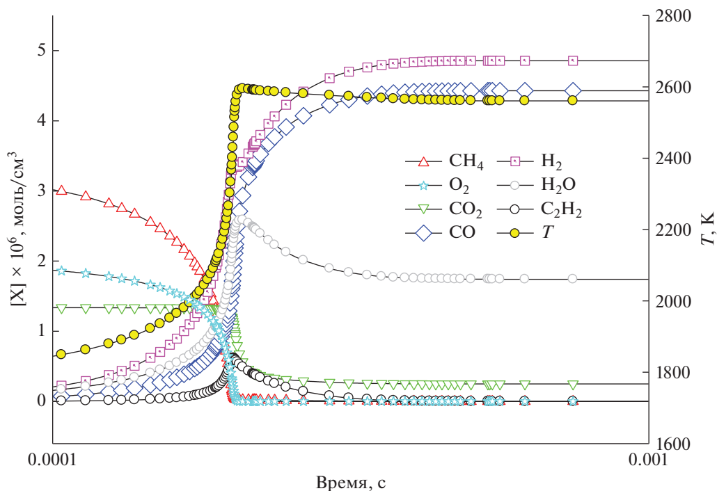
Рис. 4. Расчет изменения концентрации \text{CH}_4 , \text{CO}_2 , \text{CO} , \text{H}_2 , \text{H}_2\text{O} , \text{C}_2\text{H}_2 , \text{O}_2 и температуры при T_{50} = 1800 \text{ K} , P_{50} = 1 \text{ бар} и \phi = 3.33 .
