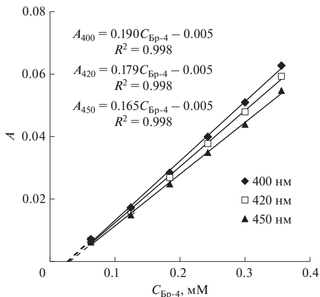
Рис. 3. Зависимости оптической плотности предельно разбавленных прямых наноэмульсий Бридж L4 от его концентрации при длинах волн 400, 420 и 450 нм.
