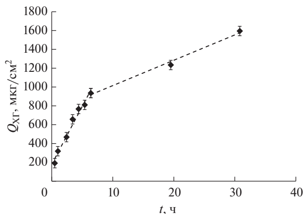
Рис. 13. Кинетика массопереноса ХГ частицами дисперсной фазы наноэмульсий Бридж Л4 ( C_{\text{Бр-4}} = 166.8 мМ).
