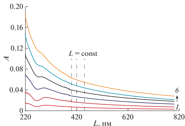
Рис. 2. Спектры A(\lambda) для наноэмульсий Бридж L4 с различными его концентрациями (через 14 дней): 1 – 0.063; 2 – 0.124; 3 – 0.184; 4 – 0.243; 5 – 0.300 и 6 – 0.356 мМ.
