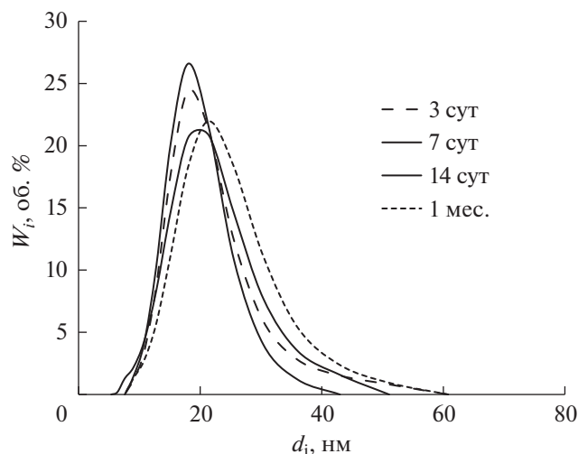
Рис. 6. Дифференциальные кривые распределения частиц по размерам для наноэмульсий Бридж L4 ( C_{\text{Бр-4}} = 166.8 мМ) с ХГ при различных временах хранения (время указано в легенде).
