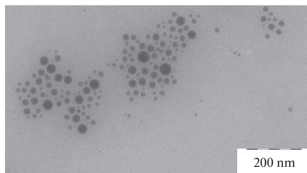
Рис. 11. Микрофотография наноземульсии Бридж L4 ( C_{\text{Бр-4}} = 166.8 \text{ мМ} ) с ХГ, полученная методом ПЭМ через 1 мес. хранения.
