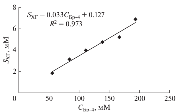
Рис. 8. Квазиравновесная изотерма солюбилизации основания хлоргексидина в наноэмульсиях Бридж L4 при 22°C.
