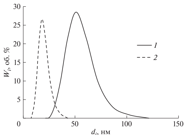
Рис. 10. Дифференциальные кривые распределения частиц по размерам наноземульсий Бридж L4 ( C_{\text{Бр-4}} = 166.8 \text{ мМ} ) без ХГ (1) и с инкорпорированным ХГ (2) через 7 сут.
