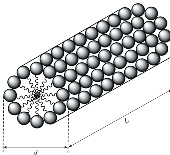
Рис. 1. Цилиндрическая мицелла.
