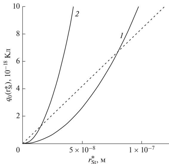
Рис. 1. Графики зависимости заряда нанобузыря q_0(r_{St}^*) от критического радиуса его слоя Штерна при концентрациях растворенной соли c_1, c_2 = 3, 8 моль/м 3 (сплошные кривые: слоя Штерна при концентрациях растворенной соли c = 3 (кривая 1) и 8 моль/м 3 (кривая 2). Штриховая линия: зависимость заряда объемного нанобузыря с термически устойчивым слоем Штерна q_{0T}(r_{St}) от его радиуса r_{St} .
