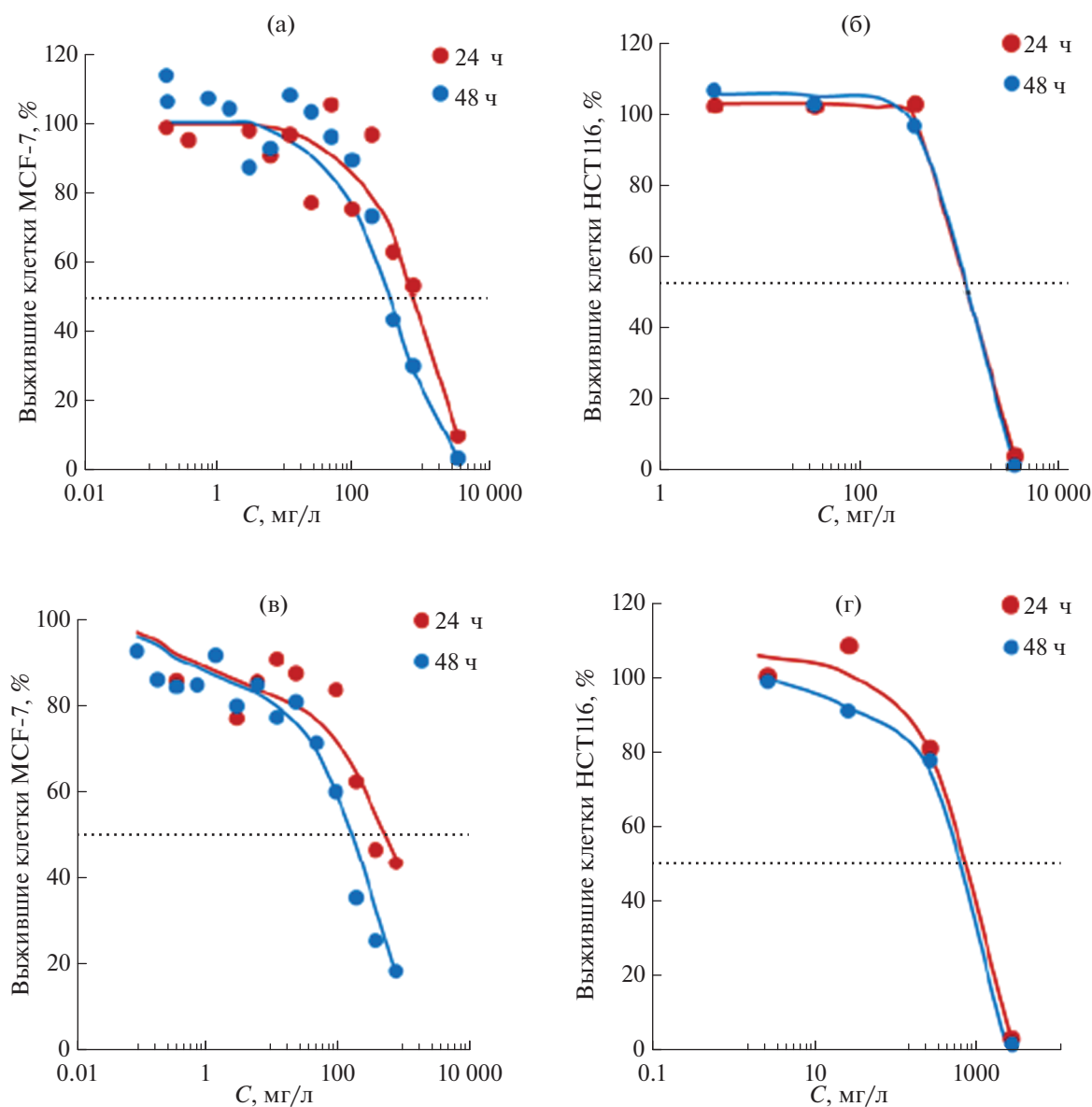
Рис. 4. Зависимости доли выживших клеток MCF-7 (а, в) и HCT 116 (б, г) от концентрации НЭ (а, б) и ТЛН (в, г). Диаметр капель в НЭ – 50 нм, ТЛН – 30 нм.
