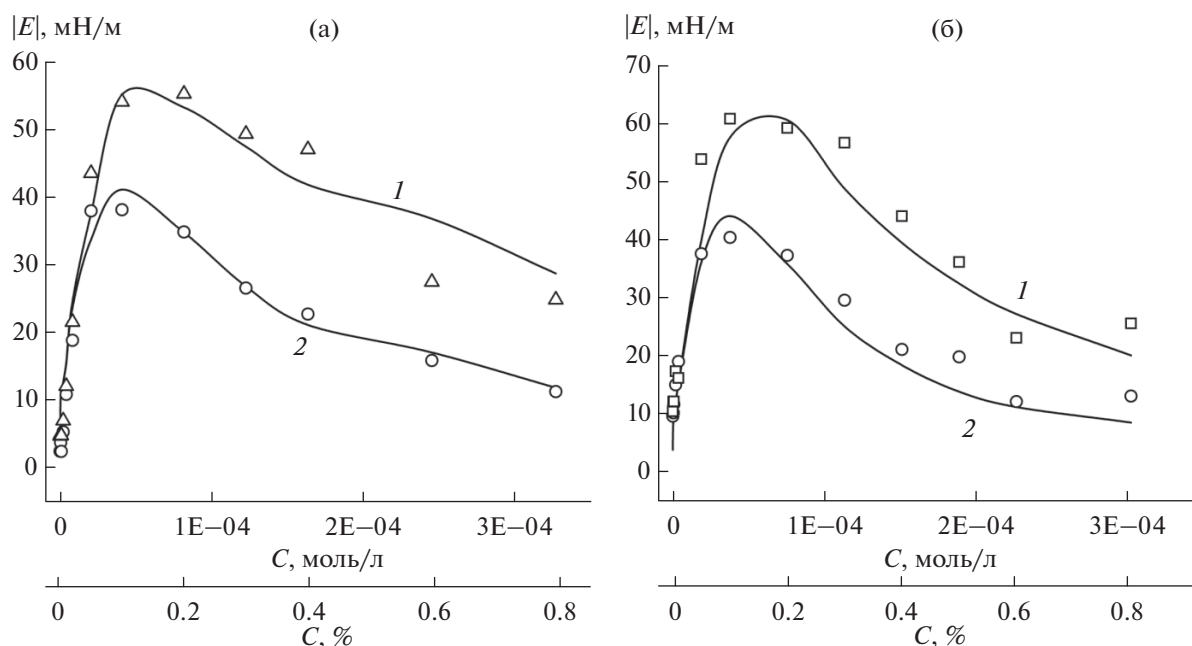
Рис. 4. Изменение величины модуля вязкоупругости от концентрации растворов гуматов натрия: (а) — ГНГК + мочевины + ПЭГ-6000; (б) — ГНГК + циангуанидин + ПЭГ-6000; 1 f=0.1 Гц; 2 f=0.01 Гц. Маркеры — экспериментальные результаты, линии — расчетные кривые. Пояснения в тексте.
