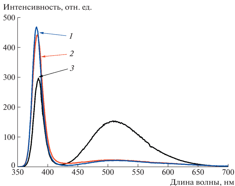
Рис. 2. Спектры ФЛ нанолистов (1), наностенок (2) и наногребенок (3).
