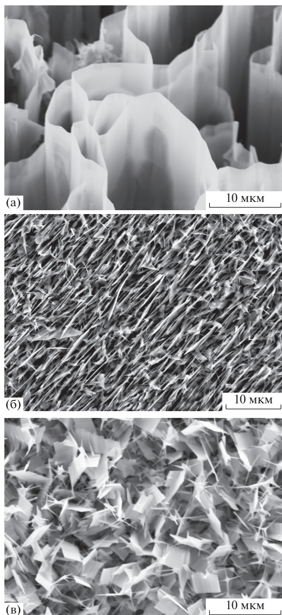
Рис. 1. РЭМ-изображения массивов наноструктур с морфологией наностенок (а), нанолистов (б) и наногребенок (в). Снимок (а) сделан под углом 45^\circ к подложке; снимки (б) и (в) – параллельно плоскости подложки.
