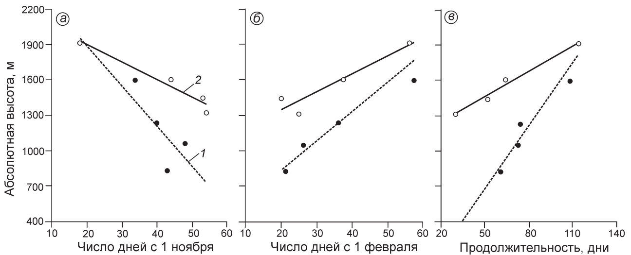
Рис. 3. Связь начала (а), конца (б) и продолжительности (в) дней с ледовыми явлениями с абсолютной высотой по наблюдениям на гидрологических постах на реках:
