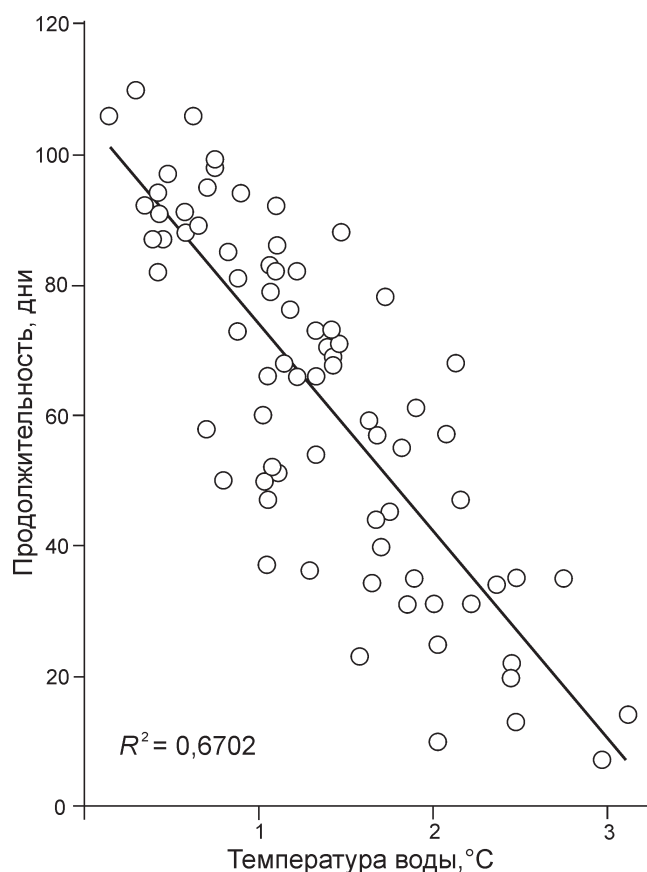
Рис. 4. Корреляционная связь между средней зимней температурой воды и продолжительностью ледовых явлений на р. Марц–п. Туманян за 1939–2018 гг. Fig. 4. Correlation between the average winter water temperature and the duration of ice phenomena on Marts river–p. Tumanyan for 1939–2018
