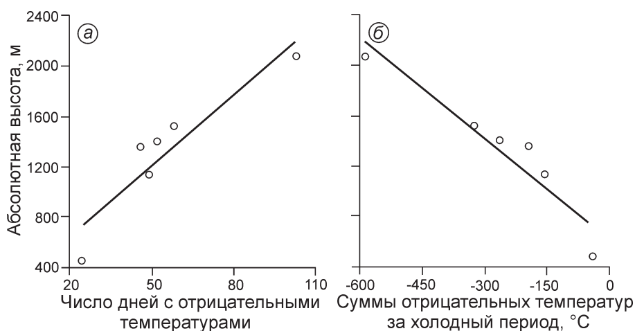
Рис. 2. Зависимость числа дней с отрицательными температурами (а) и сумм отрицательных температур воздуха (б) от абсолютной высоты местности в 1964–2018 гг.
