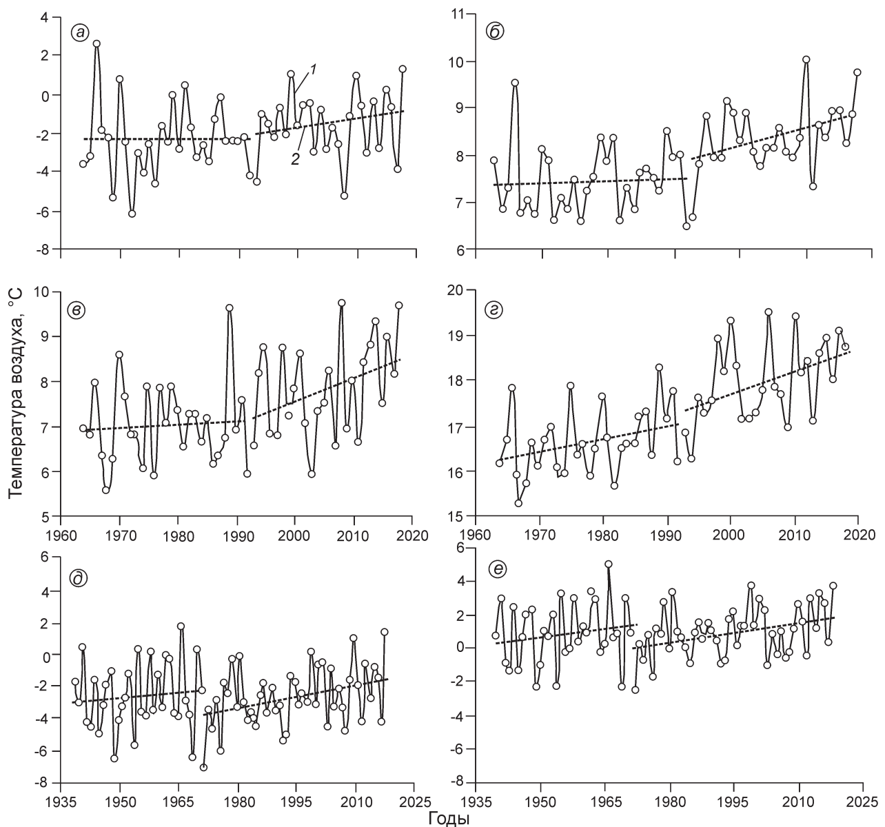
Рис. 6. Многолетние изменения средней температуры воздуха в бассейне р. Дебед: a – за декабрь–февраль; б – за год; в – за март–май; г – за июнь–август; то же за декабрь–март для МС на разных высотах: д – Ташир, 1507 м; е – Одзун, 1105 м. 1 – межгодовые колебания температур; 2 – линии трендов Fig. 6. Long-term changes of average air temperature in the Debed basin: a – for December–February; б – for year; в – for March–May; г – for June–August; the same for December–March for stations at different heights: д – Tashir, 1507 m; е – Odzun, 1105 m. 1 – interannual fluctuations; 2 – trend lines
