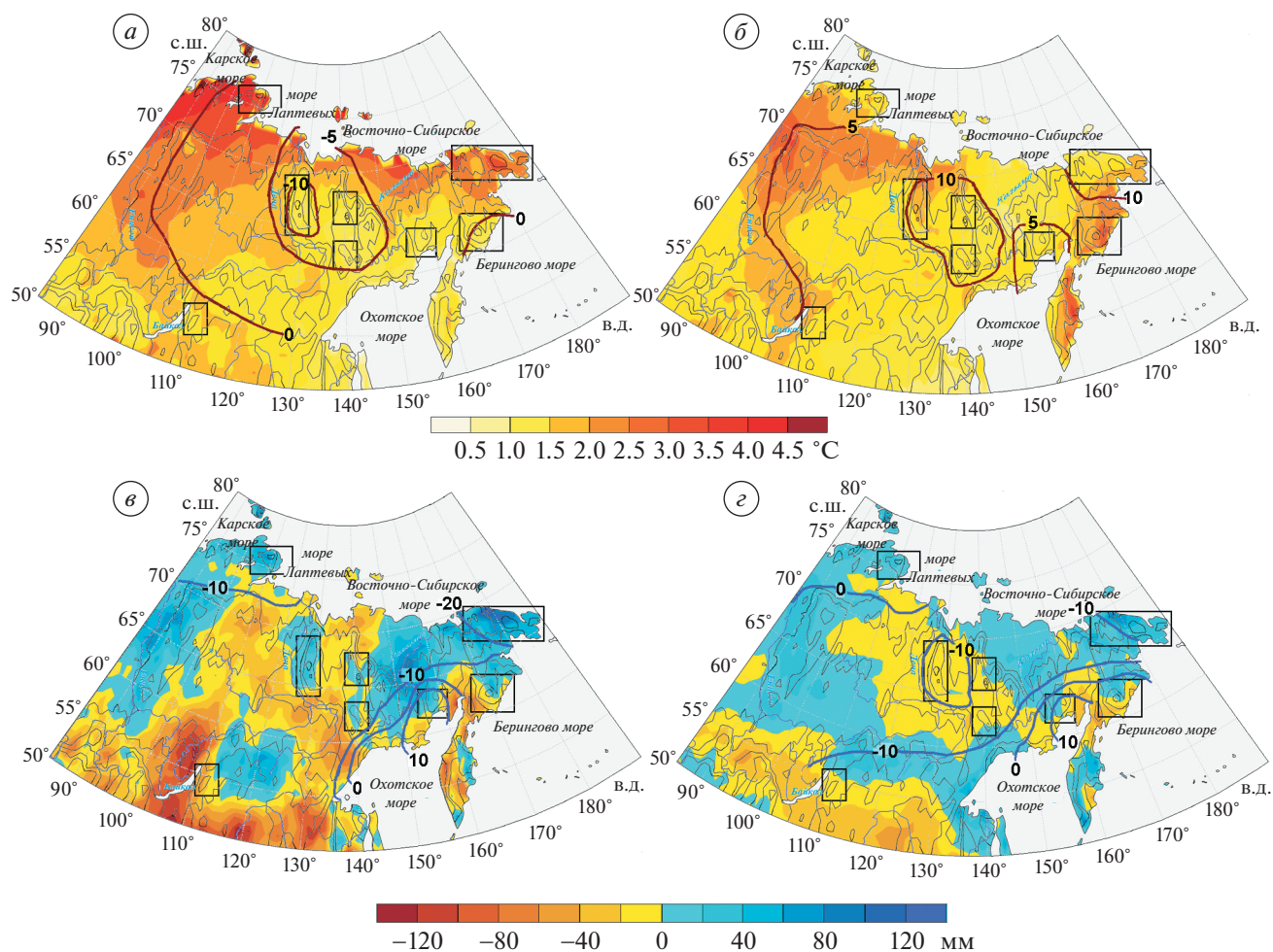
Рис. 4. Тренды параметров (цветная заливка) за 55 лет (1966–2021 гг.): (а) температура за год, °С; (б) температура за летний период, °С; (в) осадки за год, мм; (г) осадки за холодный период, мм. Изолиниями обозначена ошибка тренда (%) по данным реанализа ERA5–Land относительно стационарных наблюдений. Серыми изолиниями показан рельеф, прямоугольниками – исследуемые горные районы.
