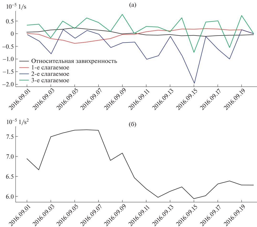
Рис. 8. Изменение со временем относительной завихренности поля скорости и слагаемых уравнения (2.1) (а) и квадрата частоты плавучести (б) на горизонте 200 м в точке (38.82° в.д., 43.83° с.ш.).
