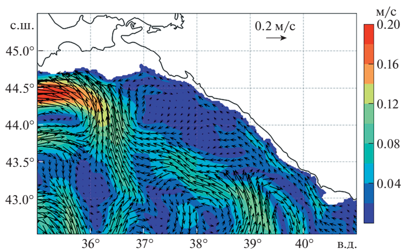
Рис. 2. Модельное поле течений в северо-восточной части Черного моря 4 сентября 2016 г. на горизонте 200 м.
