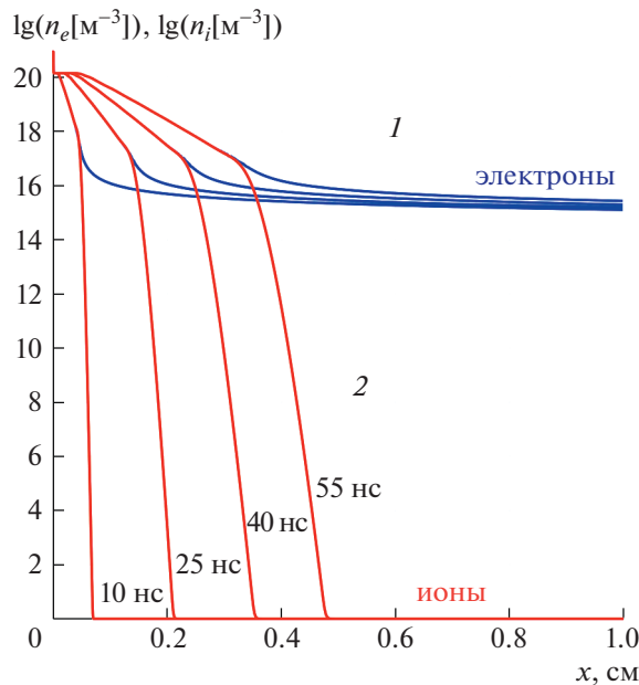
Рис. 2. Пространственно-временная картина изменения электронной (кривые 1) и ионной (кривые 2) концентрации в логарифмическом масштабе в моменты времени t = 10, 25, 40 и 55 нс.
