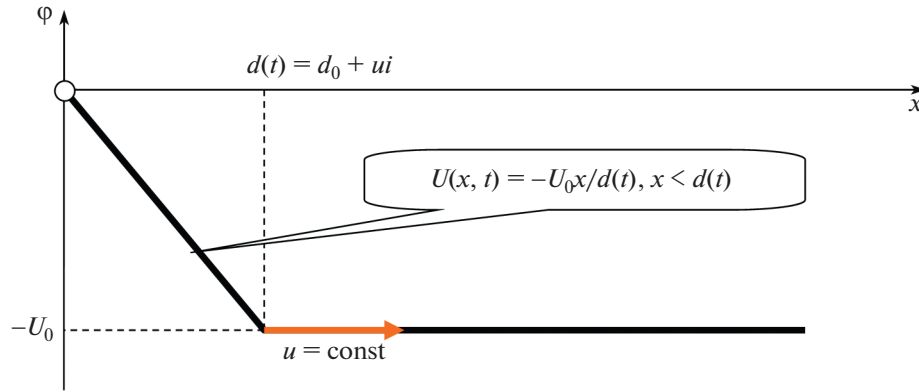
Рис. 3. Схематическое изображение движения положительно заряженной частицы в потенциальной яме, перемещающейся с постоянной скоростью.
