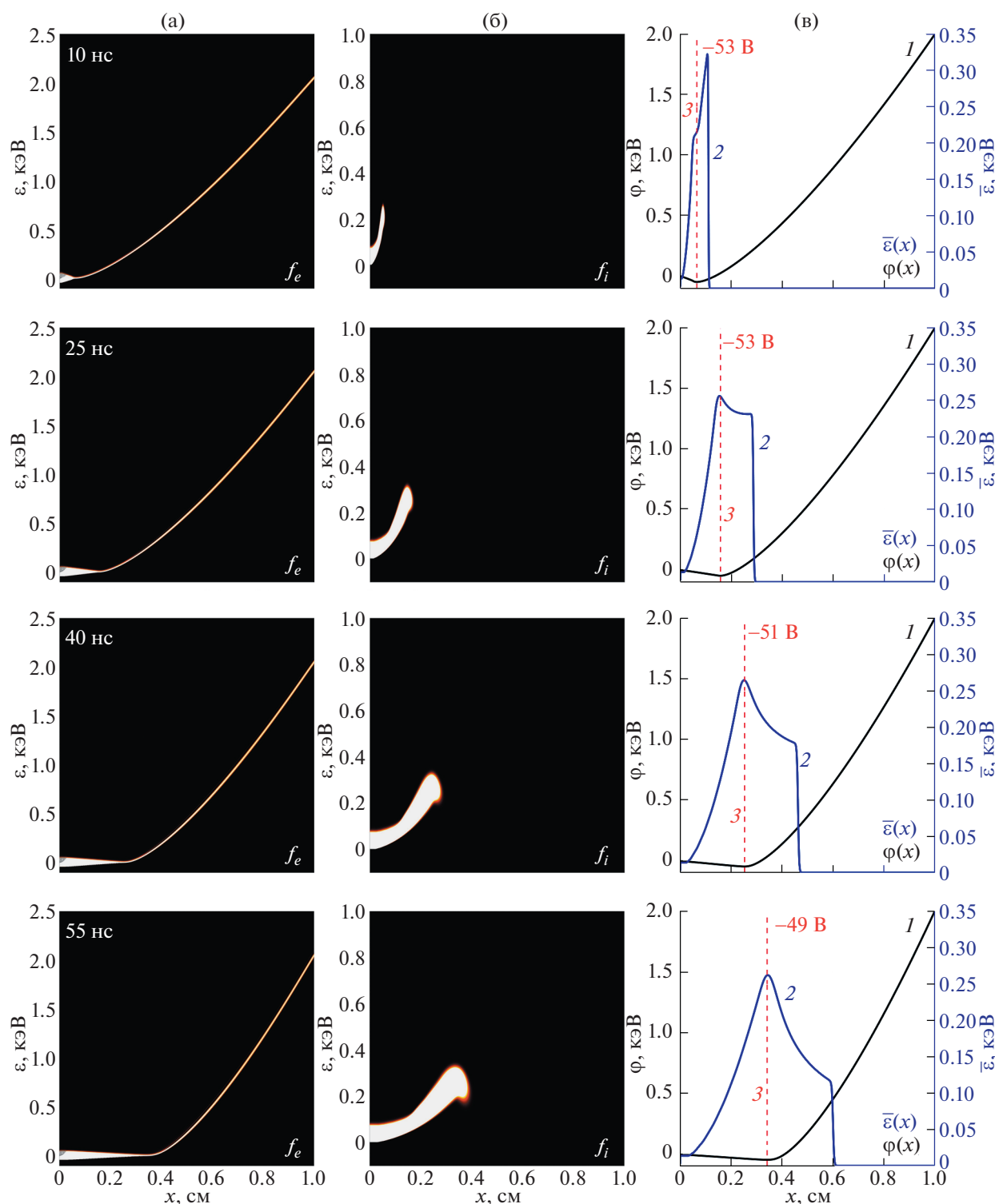
Рис. 1. Графики плотности ФРЭ (столбец А), ФРИ (столбец Б) и пространственные распределения электрического потенциала (кривая 1, столбец В) и средней энергии ионов (кривая 2), в моменты времени t = 10, 25, 40 и 55 нс. Штриховая линия 3 указывает мгновенное положение минимума потенциала и его глубину.
