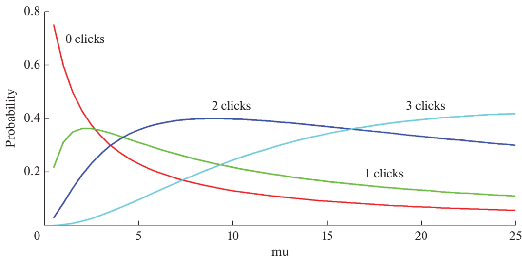
Рис. 5. Распределение числа отсчетов для тепловых состояний с различным средним числом фотонов на входе.
