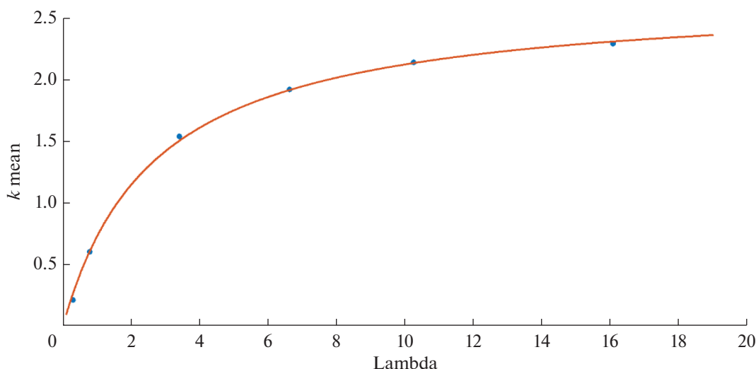
Рис. 2. Зависимость среднего числа регистрируемых фотонов от среднего числа фотонов в когерентной моде на входе.
