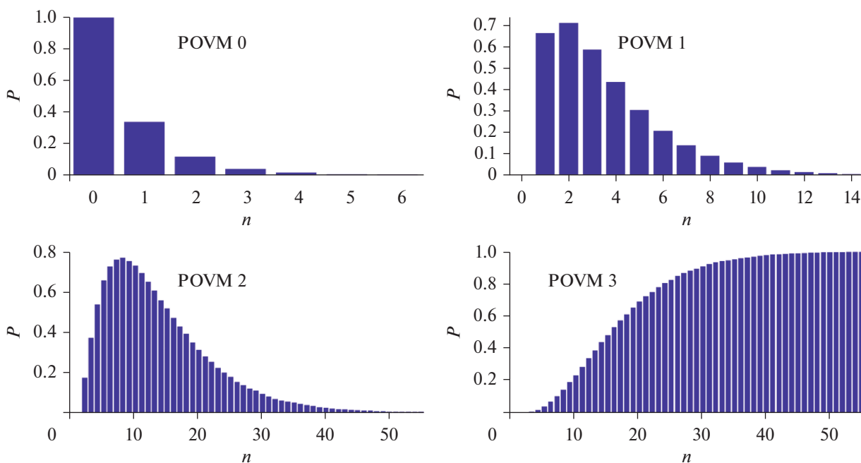
Рис. 4. POVM-элементы детектора.
