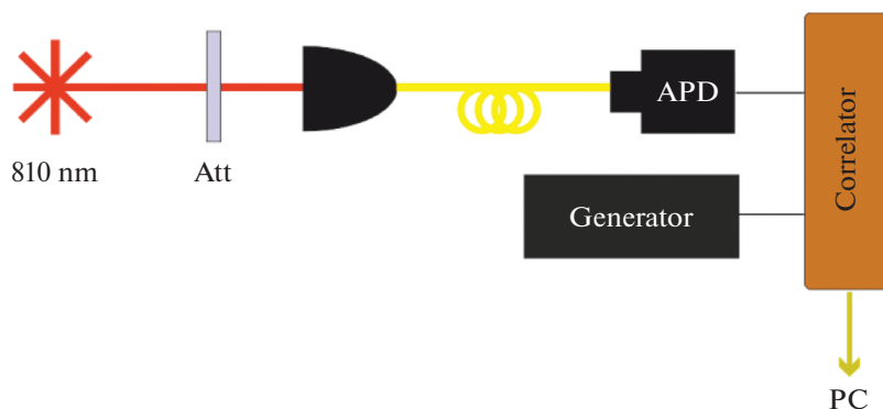
Рис. 1. Схема установки по измерению статистики фотоотсчетов. Att — поглощающий фильтр, APD — исследуемый детектор, Correlator — аналого-цифровой преобразователь (АЦП), PC — персональный компьютер.
