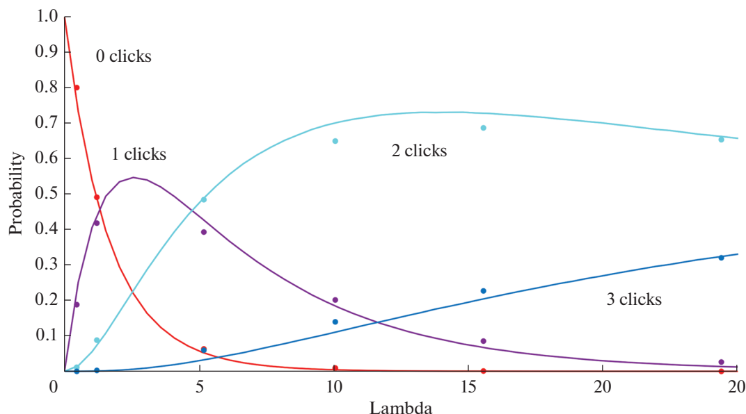
Рис. 3. Распределение числа отсчетов в приложении к томографии детекторов. На входе когерентные состояния с различным средним числом фотонов. Сплошные кривые — теория, точки — эксперимент.
