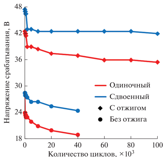
Рис. 7. Зависимость напряжения срабатывания от числа циклов коммутации.
