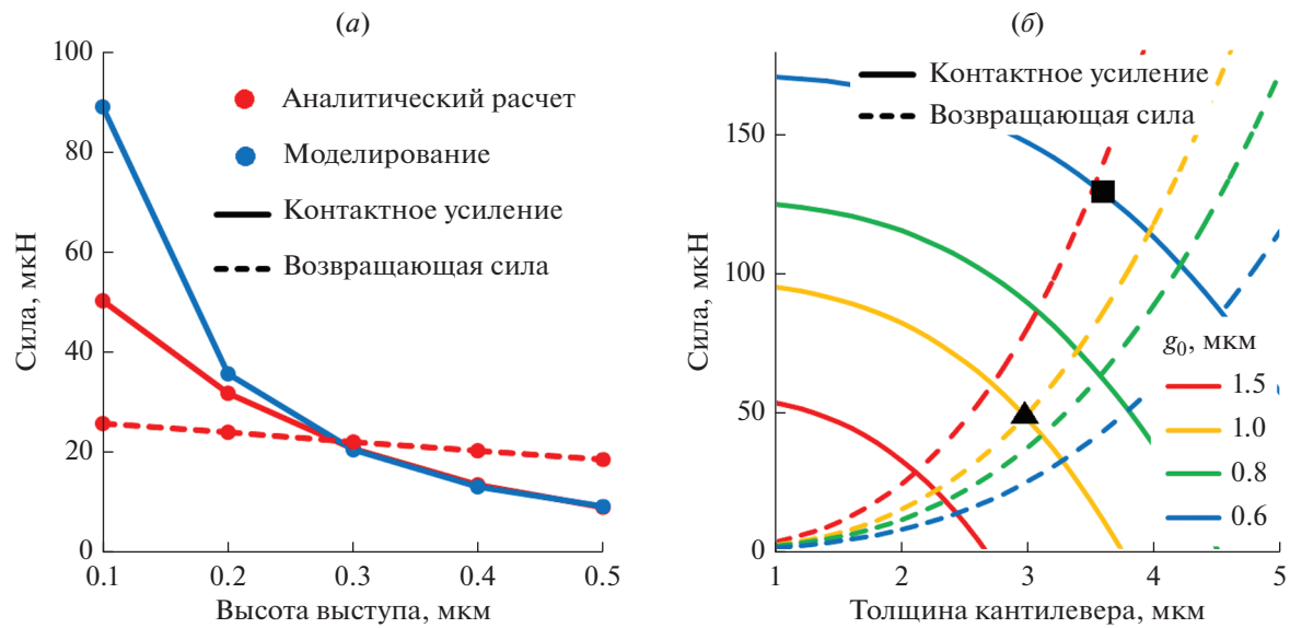
Рис. 2. Зависимость контактной и возвращающей силы от высоты контактного выступа (а) и толщины кантилевера при разных зазорах (б).
