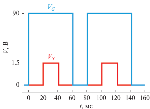
Рис. 5. Управляющее и входное напряжение.
