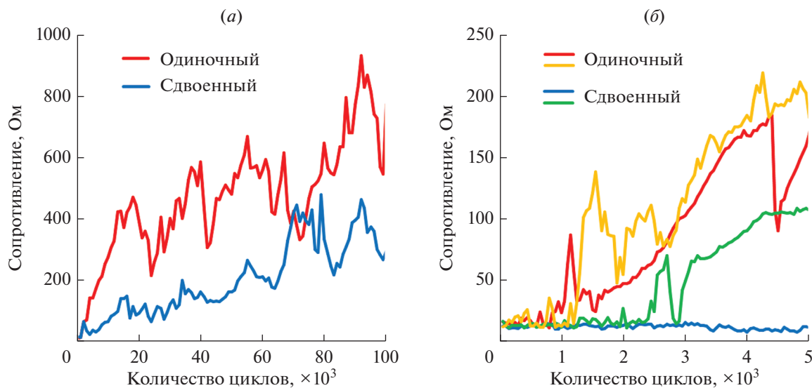
Рис. 8. Зависимость контактного сопротивления от числа циклов коммутации: (а) усредненные данные; (б) данные для четырех образцов.
