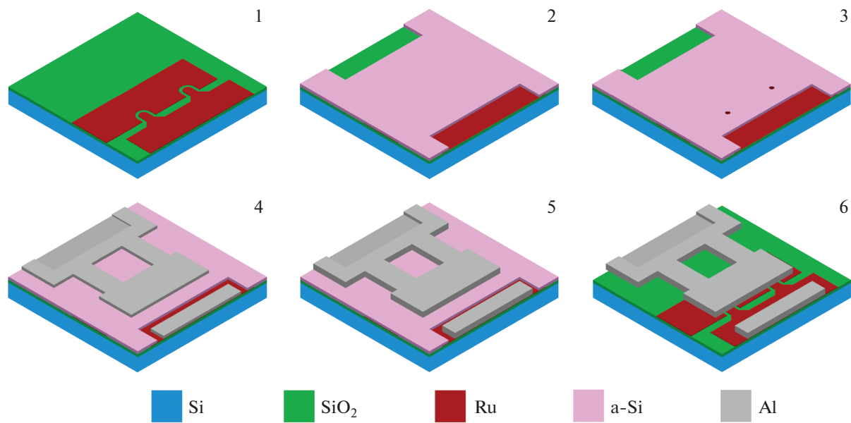
Рис. 3. Этапы изготовления переключателя.
