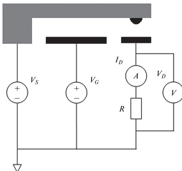
Рис. 4. Схема подключения приборов к образцу.
