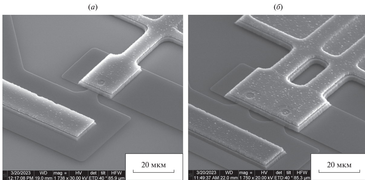
Рис. 6. СЭМ-изображения переключателей с одиночным (а) и двойным кантилевером (б).
