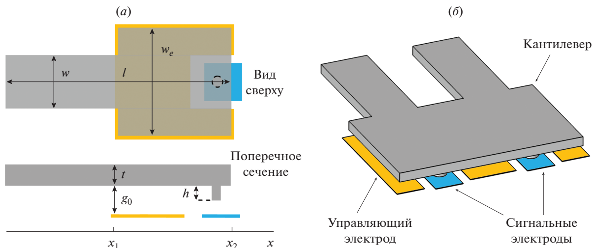
Рис. 1. МЭМС-переключатель на основе кантилевера: (а) вид сверху и поперечное сечение; (б) трехмерный вид двойной конструкции.
