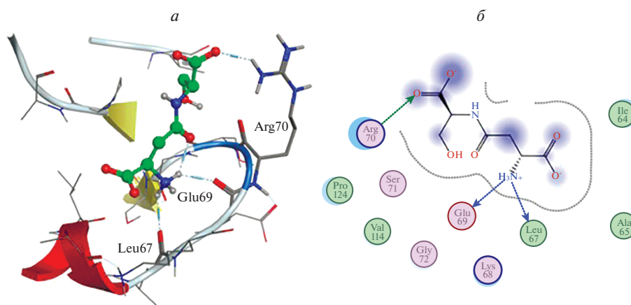
Рис. 2. Взаимодействие пептида DS с гистоном H1.3 в трехмерном (а) и двумерном (б) изображении.
