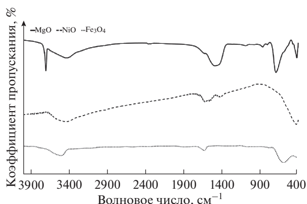
Рис. 1. FTIR-спектры наночастиц MgO, NiO и Fe 3 O 4 .
