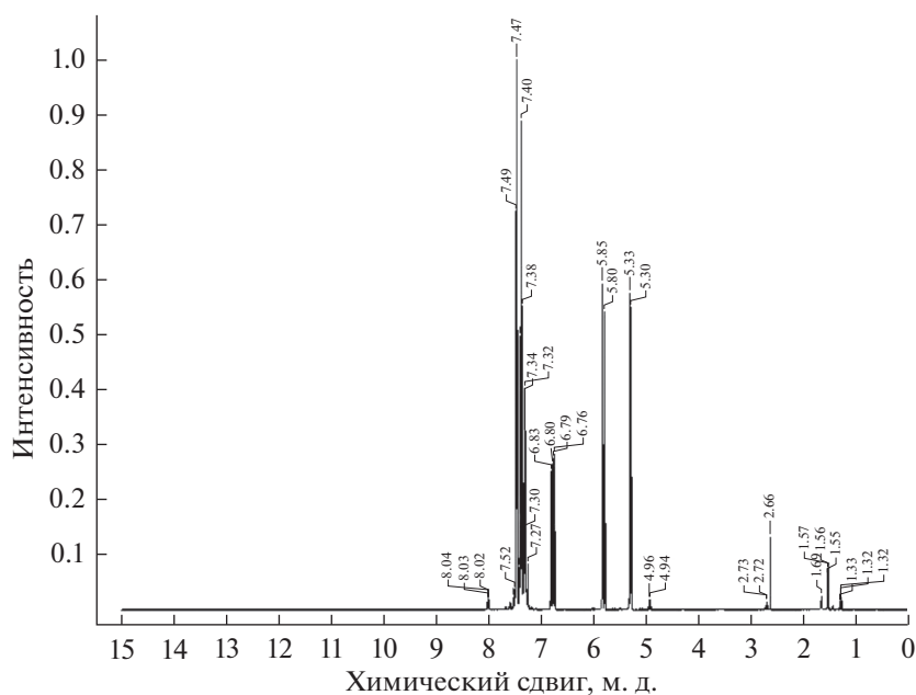
Рис. 2. ПМР-спектр ацетофенона с катализатором маггемит.
