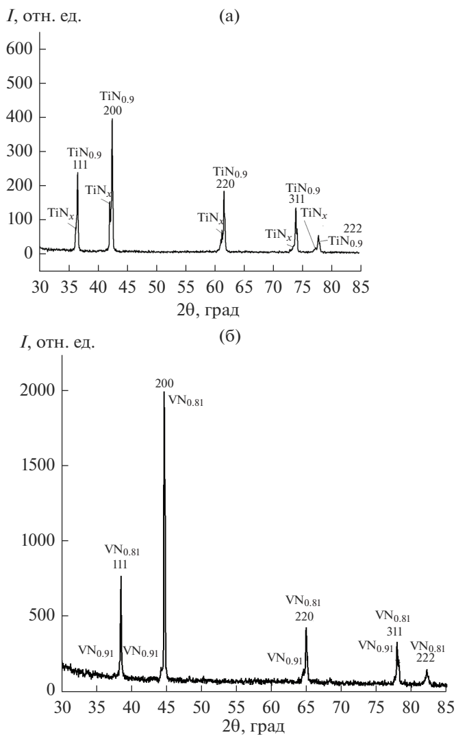
Рис. 7. Порошковые рентгеновские дифрактограммы Ti (а) и V (б), азотированных в течение 300 мин.
