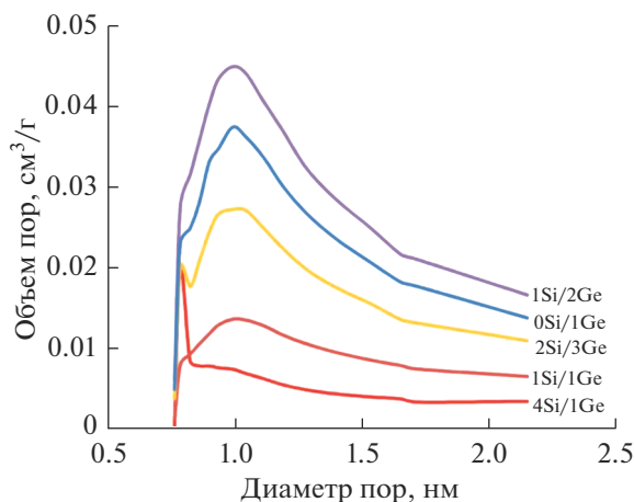
Рис. 4. Распределение микропор по размерам в пористых материалах, полученных из стекол системы \text{Na}_2\text{O}-\text{B}_2\text{O}_3-\text{SiO}_2-\text{GeO}_2 .
