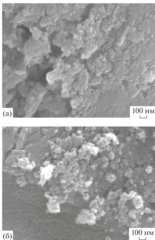
Рис. 1. Микрофотографии пористых стекол 1Si/1Ge (а), 1Si/2Ge (б).
