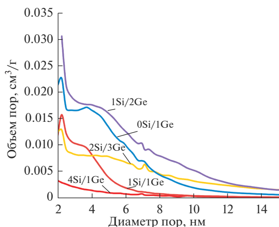
Рис. 3. Распределение мезопор по размерам в пористых материалах, полученных из стекол системы \text{Na}_2\text{O}-\text{B}_2\text{O}_3-\text{SiO}_2-\text{GeO}_2 .
