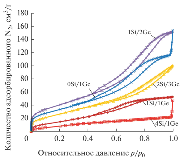
Рис. 2. Изотермы адсорбции–десорбции азота.
