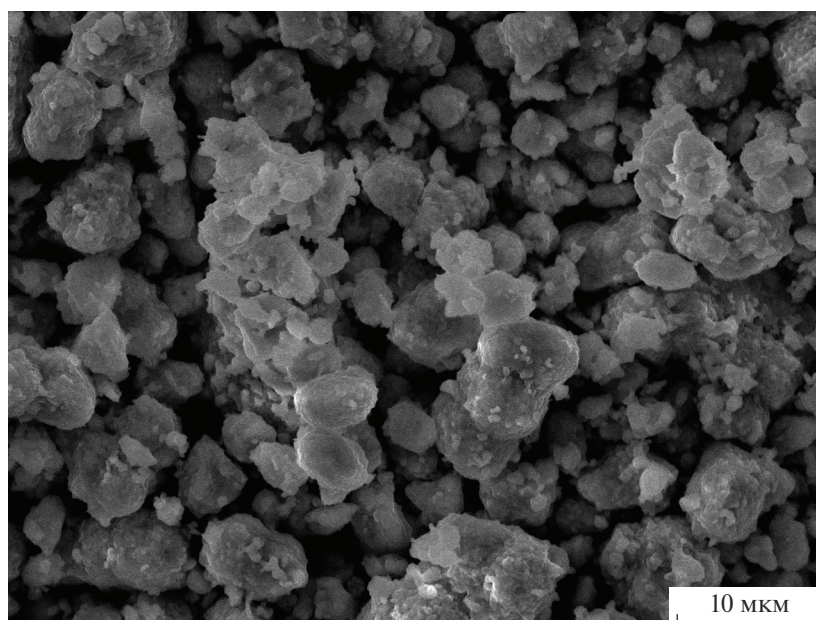
Рис. 1. Микроструктура конгломератов порошков \text{ViFe}_2(\text{PO}_4)_3 .
