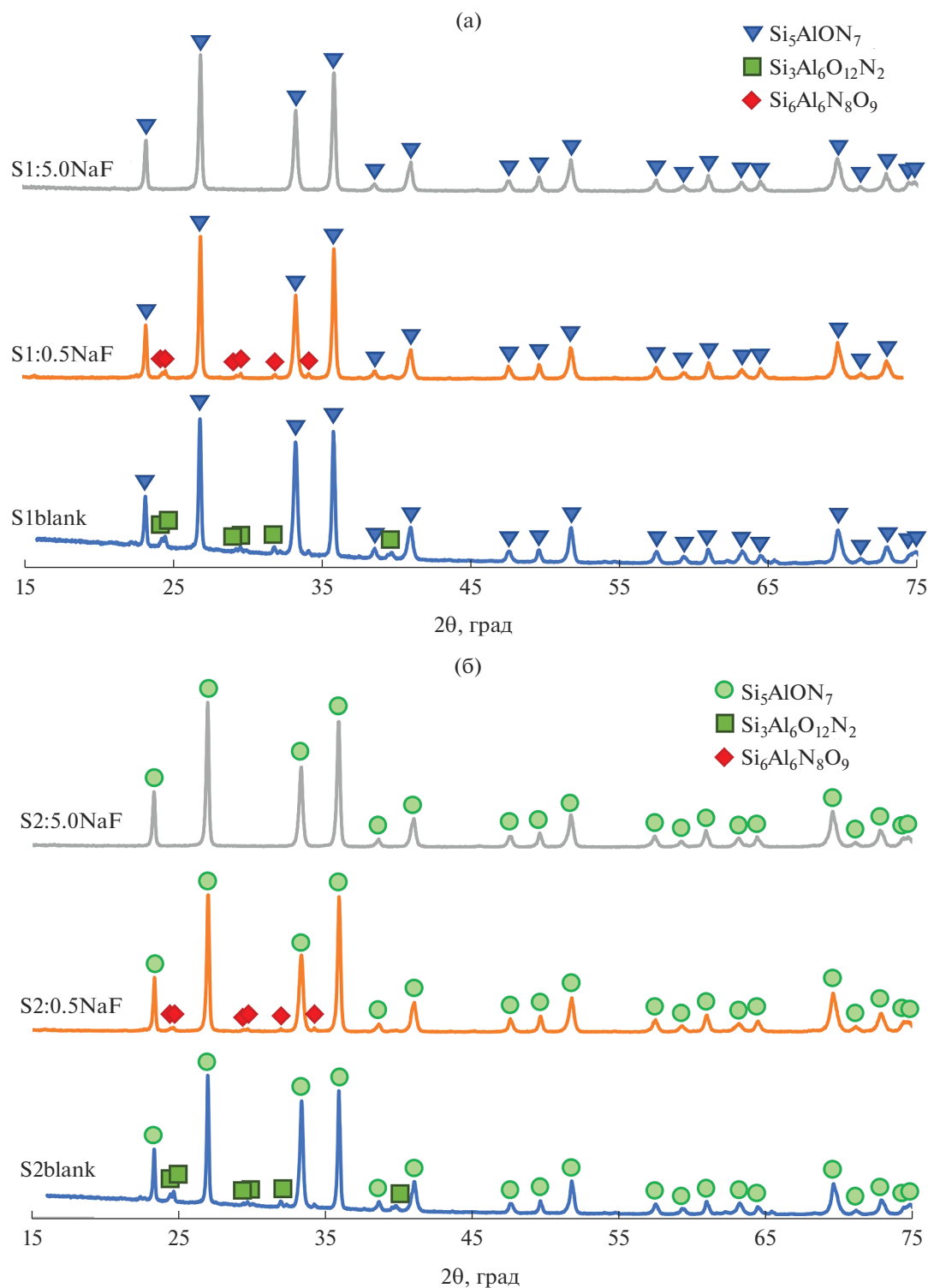
Рис. 1. Дифрактограммы образцов \beta -сиалонов S1 (а) и S2 (б) после высокотемпературного обжига без добавления NaF и с добавлением 0.5 и 5.0 мас. % NaF.
