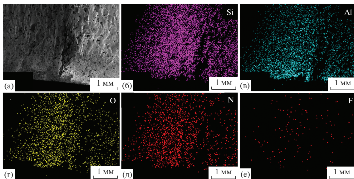
Рис. 3. РЭМ-изображение образца S1:5.0NaF (а) и результаты картирования по элементам при помощи приставки РЭДС (б–е).
