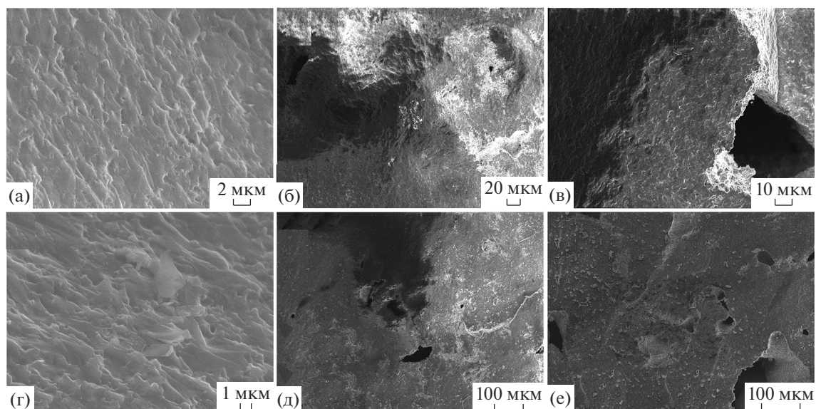
Рис. 2. РЭМ-изображения образцов S1blank (а), S1:0.5NaF (б), S1:5.0NaF (в), S2blank (г), S2:0.5NaF (д) и S2:5.0NaF (е).
