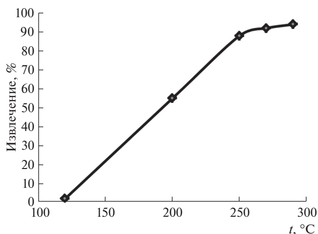
Рис. 2. Зависимость извлечения фосфора из гидроксипатита от температуры.
