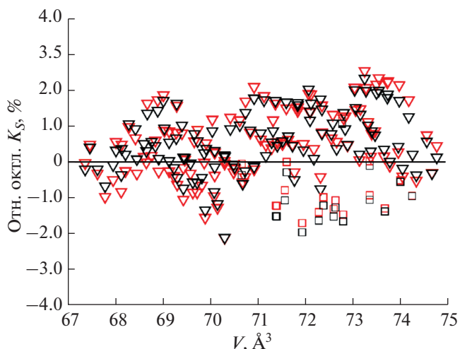
Рис. 8. Относительные отклонения адиабатического модуля упругости при давлениях до 24 ГПа и температурах от 300 до 1650 К. Красные символы – C_p -подход, черные символы – C_V -подход, треугольники – данные [14], квадраты – [48].
