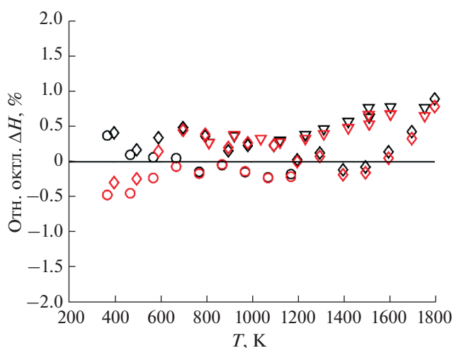
Рис. 3. Относительные отклонения между экспериментальными и расчетными значениями приращения энthalпии (круги – данные [36], треугольники – [38], ромбы – [37]) предложенных УС для MgO, P = 1 бар: красные символы – C_p -подход, черные символы – C_V -подход.
