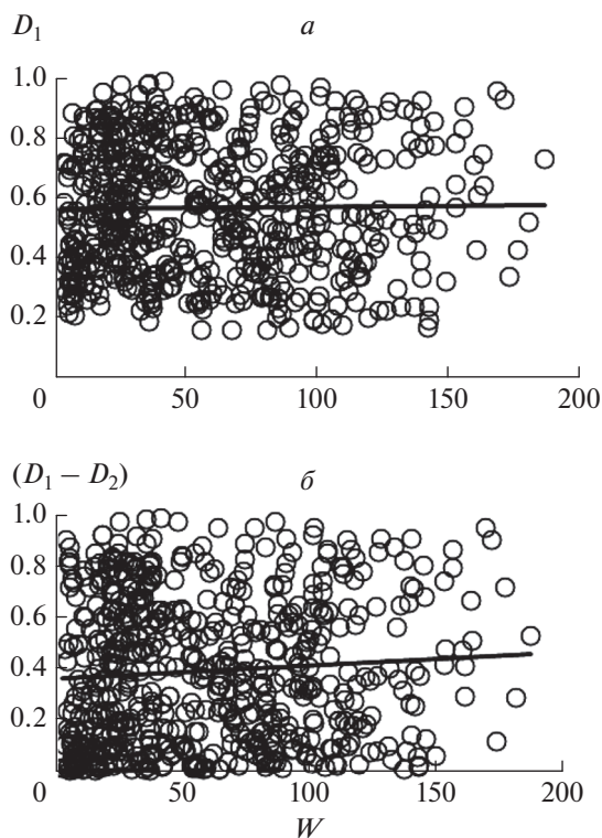
Рис. 3. Соотношения между надземной биомассой сообществ на отдельных площадках ( W ) и значениями параметров: a - D_1 (=K_1) , b - (D_1 - D_2) .
