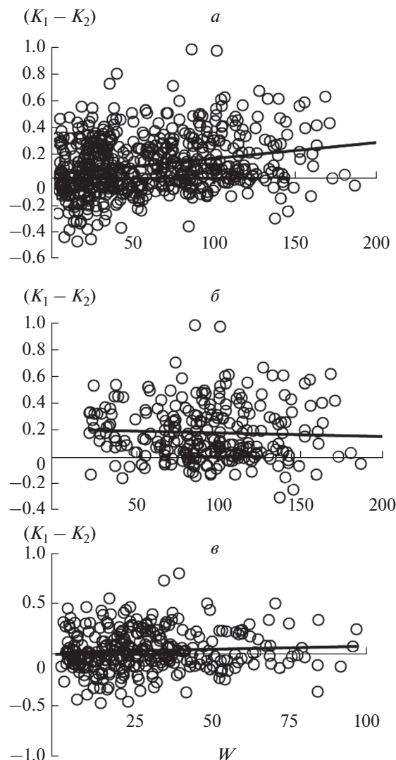
Рис. 4. Соотношения между надземной биомассой сообществ на отдельных площадках ( W ) и значениями (K_1 - K_2) . a – построены на основе всех данных, b – на основе данных по сообществам лугов и наиболее продуктивных участков степей, в – на основе данных по другим типам сообществ.
