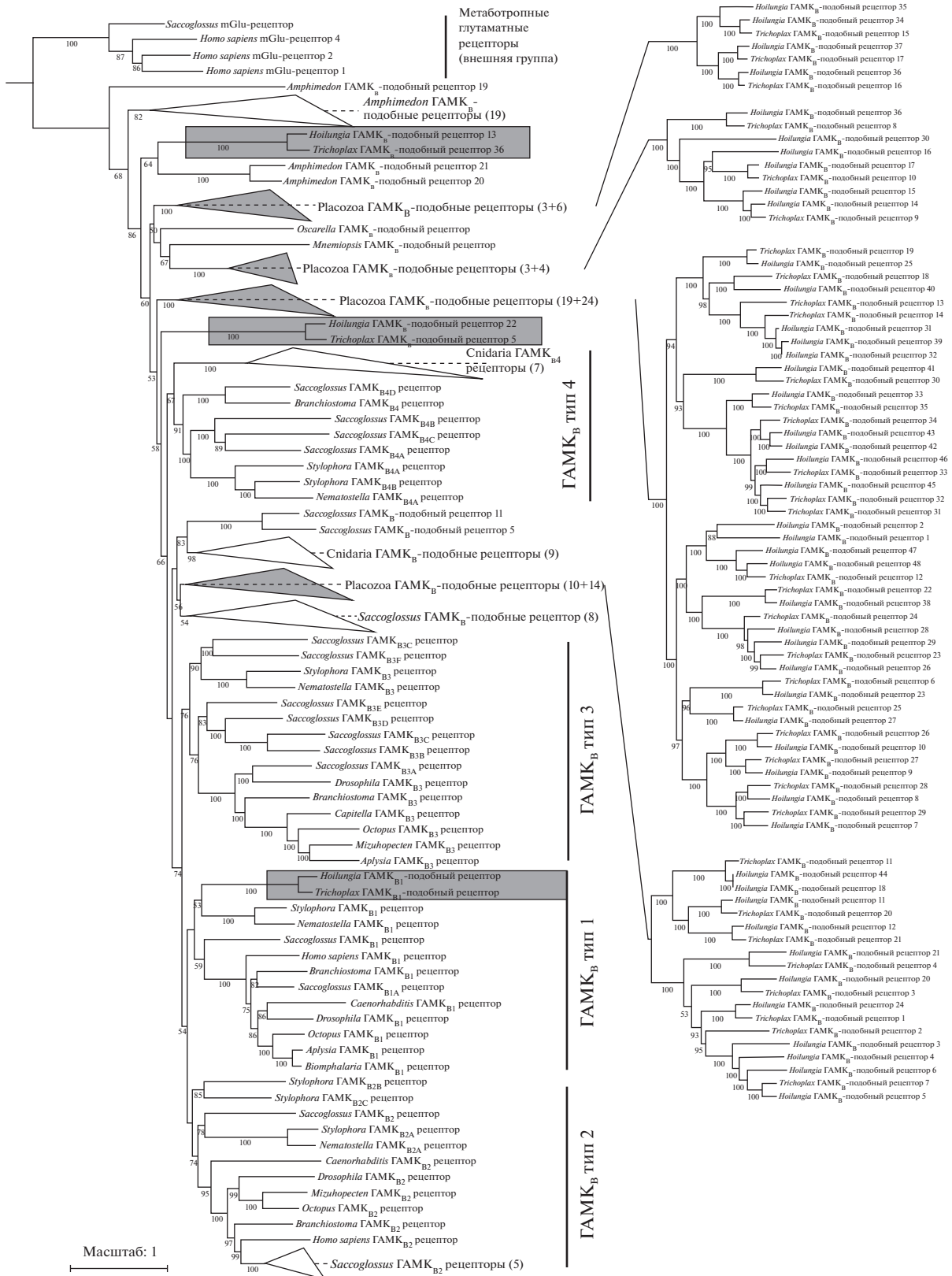
Рис. 3. Филогенетическое древо 190 метаботропных GAMK B -рецепторов животных. Древо построено методом максимального правдоподобия (Maximum Likelihood). Ветви рецепторов Placozoa выделены серым фоном. Ветви многочисленных рецепторов одного и того же организма схлопнуты в треугольники. Схлопнутые ветви рецепторов Placozoa показаны в развернутом виде в правой части рисунка. Выравнивание состояло из 6303 позиций, 1700 из них информативных.
