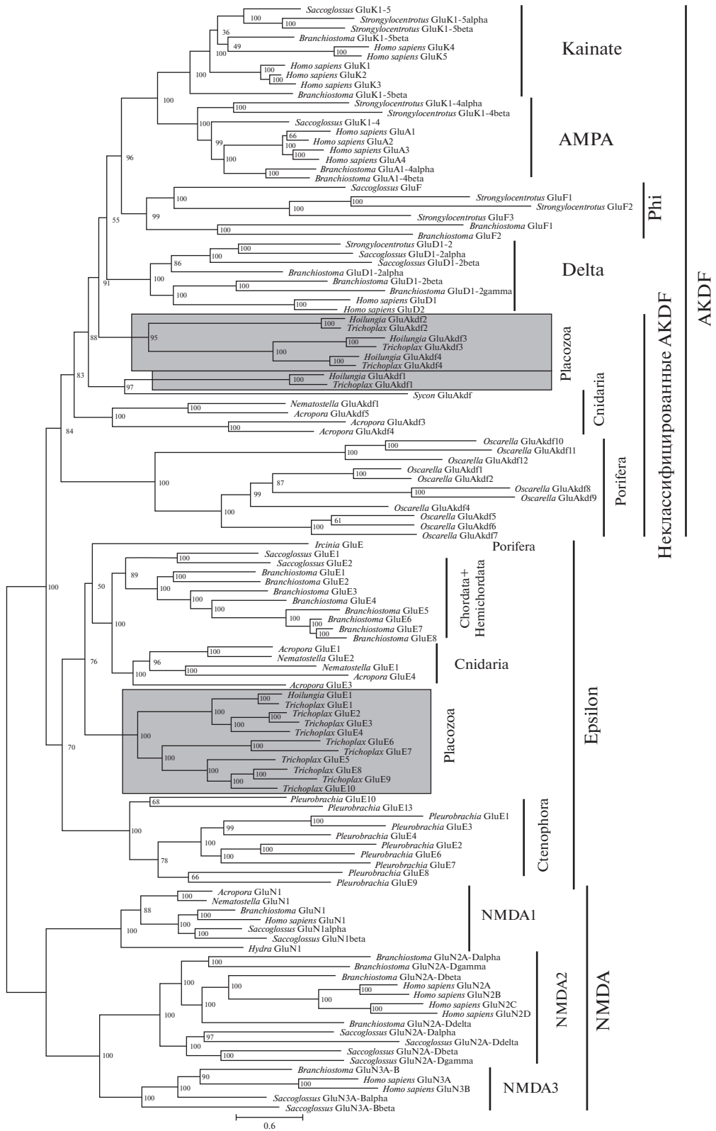
Рис. 1. Байесово филогенетическое древо 117 ионотропных глутаматных рецепторов животных. Ветви рецепторов Плацозоа выделены серым фоном. Байесовы постериорные вероятности ветвей обозначены цифрами около узлов дерева. Анализ продолжался 1.42 млн поколений до конвергенции марковских цепей, определенной с помощью программы Трасер. Выравнивание состояло из 2472 позиций, 1348 из них информативных.
