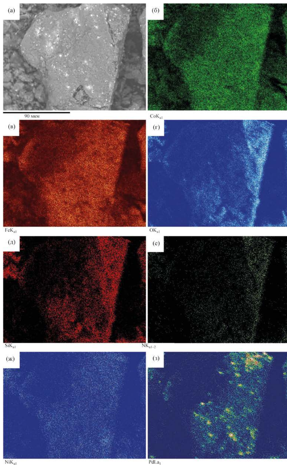
Рис. 2. СЭМ-Изображение (масштаб 90 мкм) композита Pd-Fe-Co-Ni/CoFe 2 O 4 @Si-NH 2 @Pd 2 (а) с картами распределения элементов: кобальта (б), железа (в), кислорода (г), кремния (д), азота (е), никеля (ж) и палладия (з).
