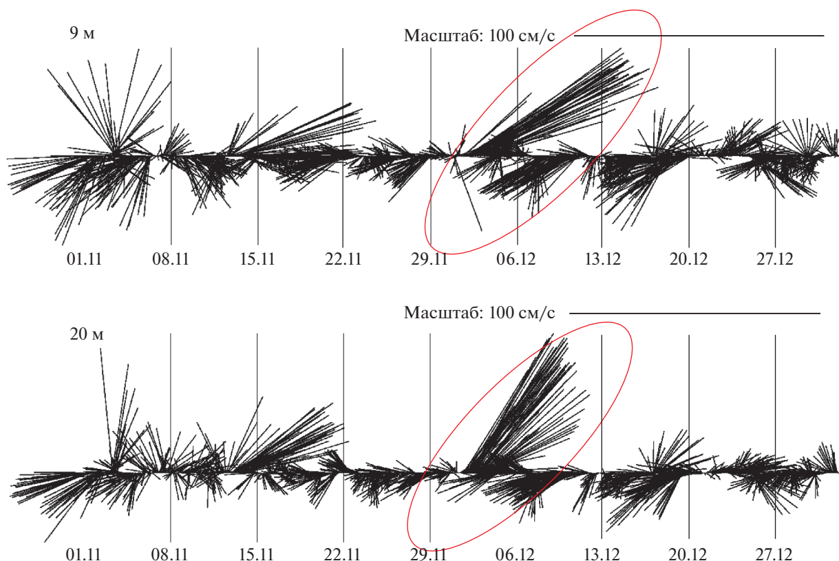
Рис. 4. Скорость течения на верхнем и нижнем горизонтах (9 и 20 м) по данным измерителей на бье 1 (залив Посыета) в ноябре–декабре 2014 г. Отмечено усиление скорости прибрежного течения 01.12.2014 г.
