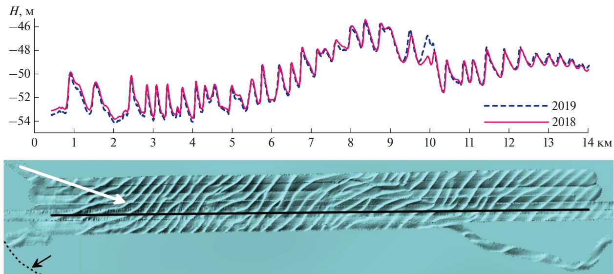
Рис. 4. Осадочные волны на полигоне 3. Снизу — акустическое изображение полигона по данным многолучевого эхолота. Белая стрелка указывает направление течения, а черная — направление на береговую линию по нормали. Сверху — профили морского дна, полученные в результате повторного картирования в 2018 и 2019 гг., черной линией снизу показано расположение профилей.
