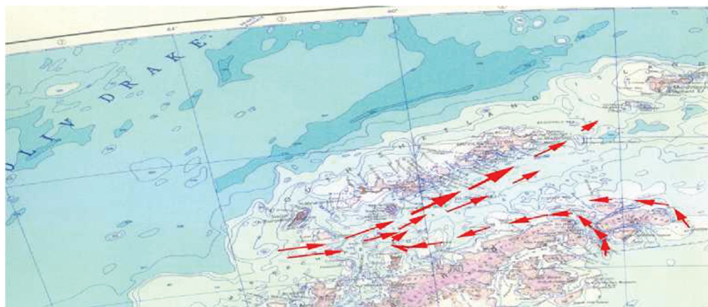
Рис. 2. Схема течений в проливе Брансфила.
