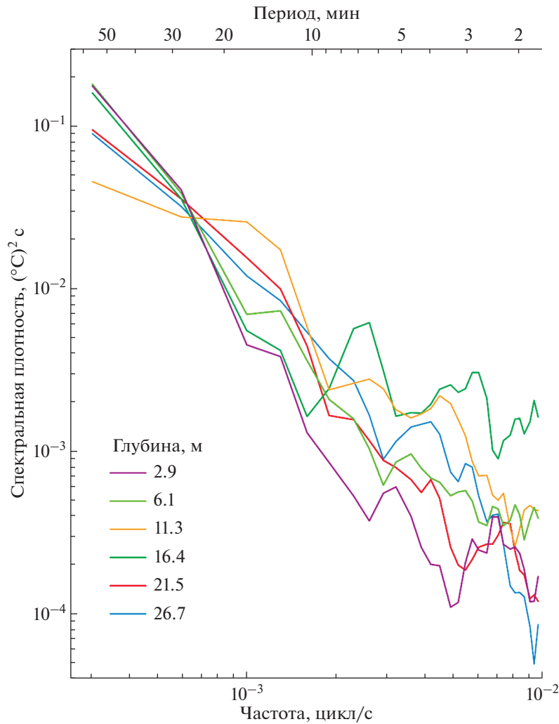
Рис. 8. Энергетические спектры колебаний температуры на 6 горизонтах измерений.
