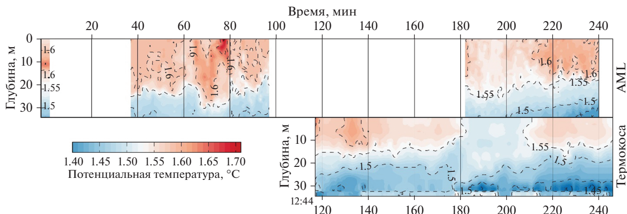
Рис. 4. Совмещенный график изменения температуры на станции 7312 по данным CTD-зонда AML Base X и датчикам термокосы 25.01.2022. По оси x дано время в минутах. Начало верхней и нижней осей соответствует времени 10:47 (начало первого тестового зондирования). По оси y дана глубина зондирования в метрах.
