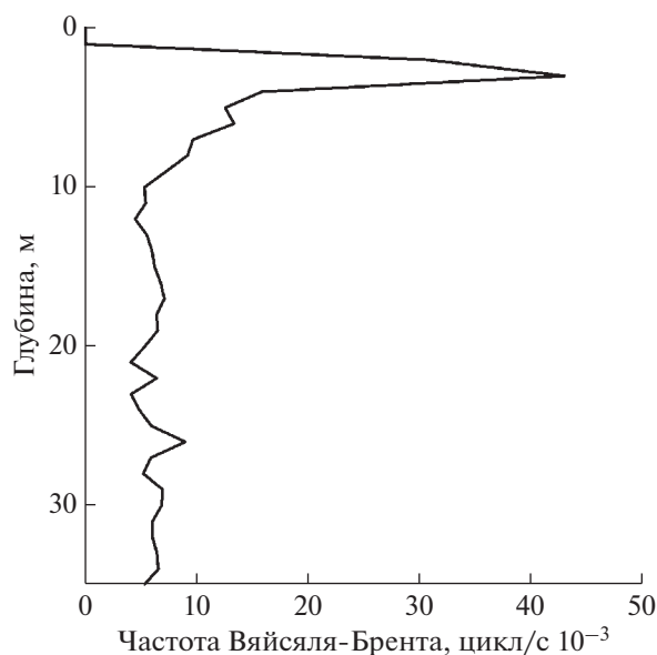
Рис. 7. Средний профиль частоты плавучести по данным STD-зондирований.
