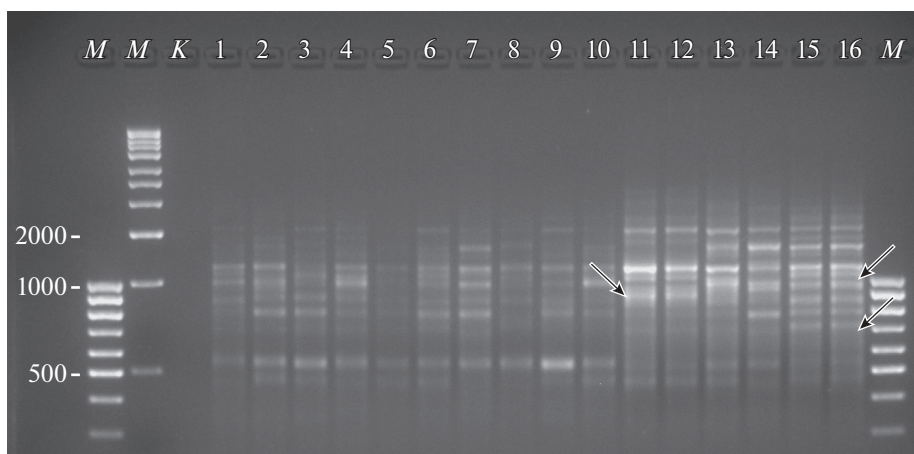
Рис. 2. ISSR-спектр разных генотипов T. suaveolens , полученный при использовании праймера UBC824. M – маркер молекулярного веса; K – отрицательный контроль; 1–10 – особи донорной популяции Озинского района Саратовской области; 11–16 – растения-регенеранты (11–13 – Var1; 14–16 – Var2). Стрелки указывают на отсутствующие у донорной популяции фрагменты.
