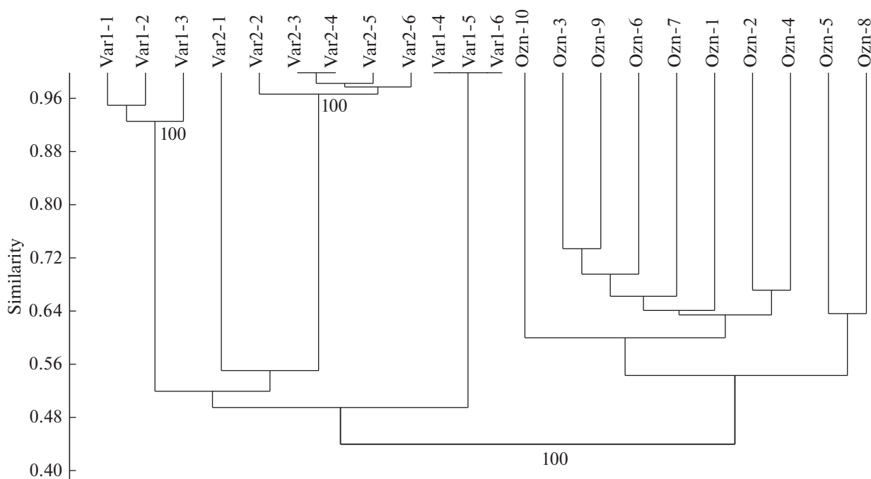
Рис. 3. UPGMA-дендрограмма, построенная на основе ISSR данных для T. suaveolens , с использованием коэффициента Жаккара. Бутстреп = 100 реплик, показана только достоверная бутстреп-поддержка – более 70%. Ozn – особи донорной популяции; Var1 – регенеранты, образованные на питательной среде с БАП 0.2 мг/л + НУК 0.5 мг/л и Var2 – регенеранты, образованные на питательной среде с БАП 0.5 мг/л + НУК 1.0 мг/л.
