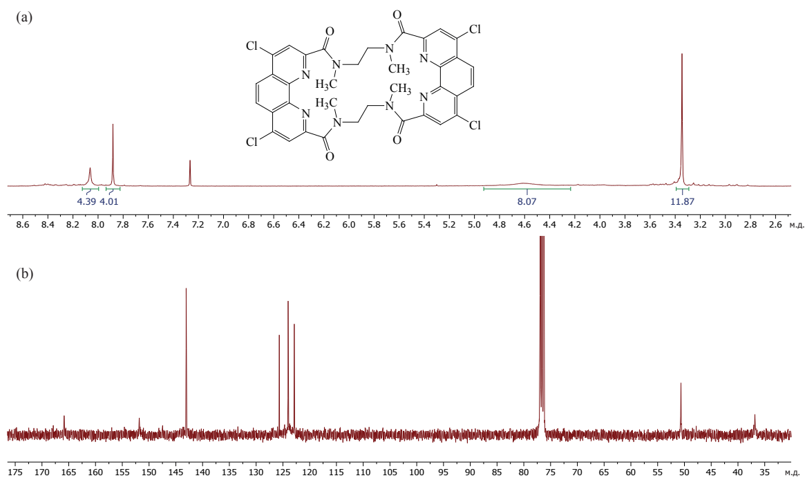
Рис. 3. Спектры ^1\text{H} -ЯМР (а) и ^{13}\text{C} -ЯМР (б) макроцикла 4 в \text{CDCl}_3 при 22°C.
