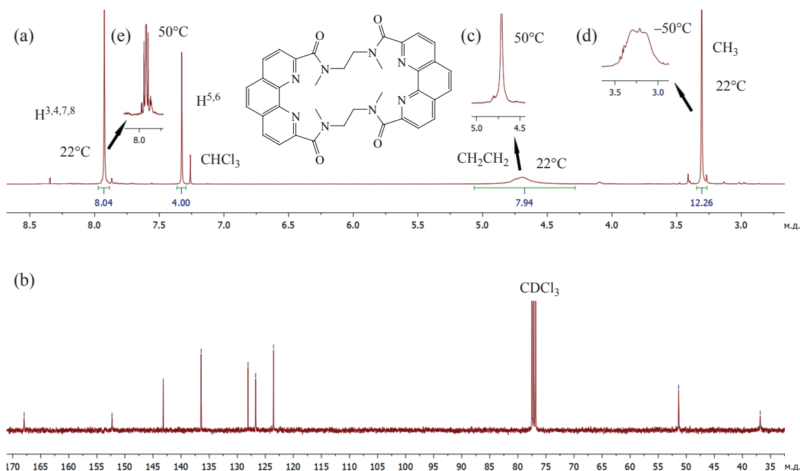
Рис. 2. Спектры ^1\text{H} -ЯМР (а) и ^{13}\text{C} -ЯМР (б) макроцикла 3 в \text{CDCl}_3 при 22°C. На врезках представлен вид сигнала \text{CH}_2 -групп при 50°C (с), вид сигнала \text{CH}_3 -групп при -50°C (д) и вид сигналов \text{H}^{3,4} и \text{H}^{7,8} при 50°C (е)
