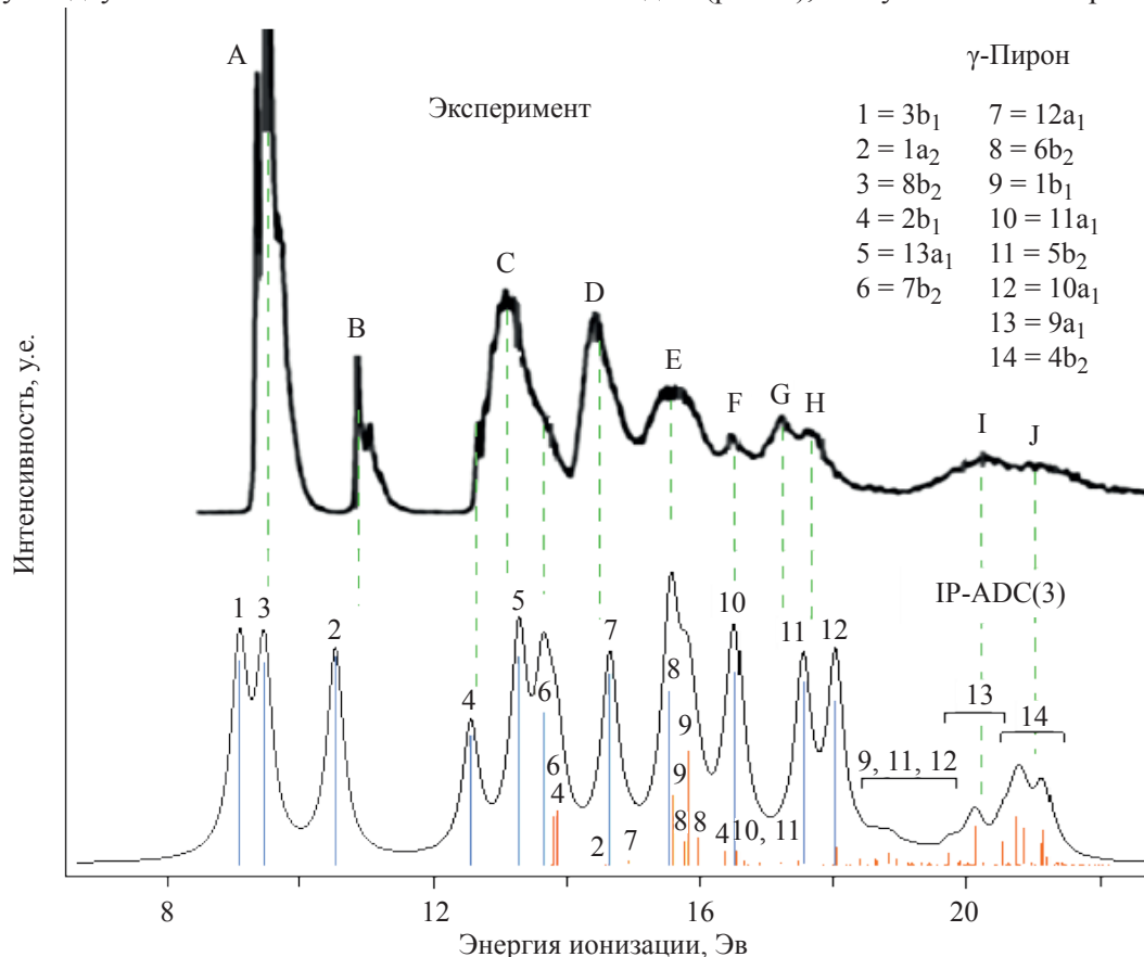
Рис. 3. Теоретический [IP-ADC(3)/aug-ss-pVTZ] и экспериментальный спектры ионизации \gamma -пирона. Теоретический спектр сдвинут на -0.30 эВ относительно экспериментального; синим обозначены вертикальные переходы, которые могут рассматриваться как основные линии (с интенсивностями P \geq 0.5 ), красным – переходы, соответствующие сателлитным линиям ( P < 0.5 )
