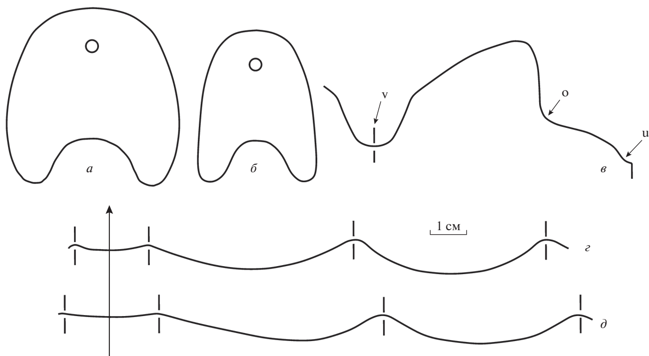
Рис. 1. Поперечное сечение, форма устья и лопастная линия Shikhanonautilus : a – поперечное сечение S. siphonoventralis Leonova et Shchedukhin, 2020, экз. ПИН, № 5668/197; б – поперечное сечение S. compressus sp. nov., экз. ПИН, № 5668/220; в – форма устья S. siphonoventralis , экз. ПИН, № 5668/198; г – перегородочная линия S. compressus sp. nov., экз. ПИН, № 5668/220; д – перегородочная линия S. siphonoventralis , экз. ПИН, № 5668/197. Обозначения: о – окулярный синус, в – вентральный (гипономический) синус, и – умбиликальный синус.
