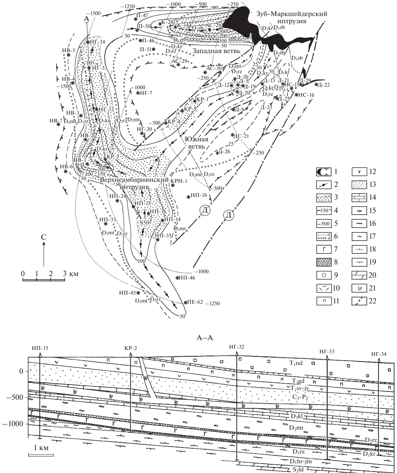
Рис. 1. Геолого-структурная схема Зубовского интрузива. 1–7 – Зубовский интрузив: 1 – выход на поверхность и граничный контур, 2 – осевые линии, 3 – ареал рудоносных ультраосновных пород и тацитовых габбро-долеритов, 4 – изопахиты, 5 – изогипсы подошвы, 6 – вмещающие породы: а – перекрывающие, б – подстилающие, 7 – положение в разрезе; 8 – контактово-метаморфический ореол; 9–12 – вулканиты: свиты – 9 – надеждинская, 10 – хаканчанская, 11 – гудчихинская, 12 – сыверминская-ивакинская; 13–20 – осадочные породы: свиты – 13 – тунгусская серия, 14 – каларгонская, 15 – мантуровская, 16 – разведочнинская, 17 – курейская, 18 – зубовская, 19 – хребтовская-ямпахтинская, 20 – силурийские отложения; 21 – Далдыканский интрузив; 22 – Далдыканский разлом и прочие дизъюнктивы.
