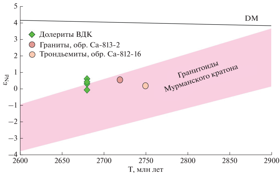
Рис. 9. Диаграмма \epsilon_{Nd} –Возраст для долеритов ВДК и вмещающих гранитоидов.
