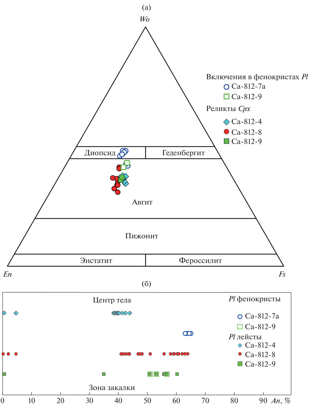
Рис. 3. Вариации составов клинопироксена и плагиоклаза в породах ВДК. (а) – положение точек составов клинопироксенов на диаграмме волластонит ( Wo )–энстатит ( En )–ферросилит ( Fs ) (Morimoto et al., 1988), (б) – вариации состава плагиоклаза, An , % – содержание анортитового минала.
