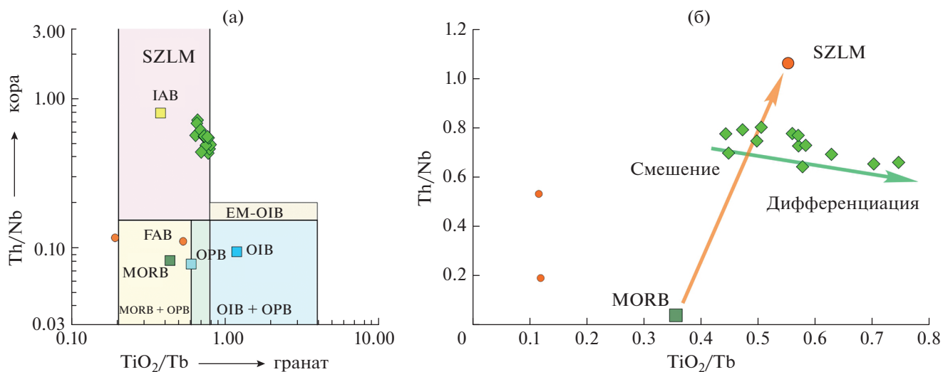
Рис. 10. (а) Положение точек составов базитов на диаграмме Пирса (Pearce et al., 2021).
