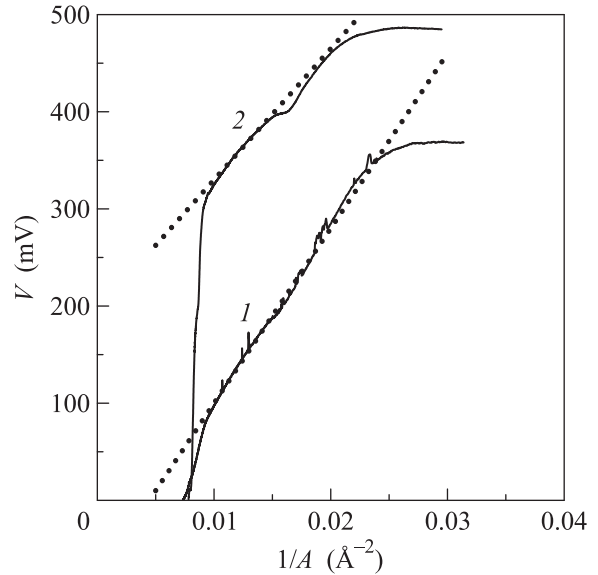
Рис. 5. Волта потенциал монослоев DMPS (см. обозначения на рис. 1), представленный в зависимости от плотности липида в монослое на поверхности соответствующих растворов (непрерывные линии). Точками показаны прямые линии, аппроксимирующие линейные участки кривых. Оценка величины эффективного дипольного момента, найденная по соотношению Гельмгольца на линейных участках кривых, составляет 0.48 и 0.38 Дебая для кривых 1 и 2, соответственно
