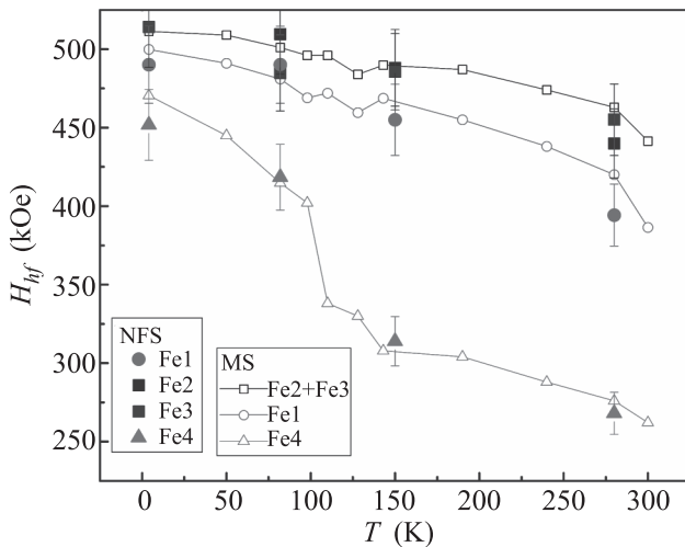
Рис. 3. (Цветной онлайн) Температурная зависимость сверхтонкого поля H_{hf} ультрамалых наночастиц \epsilon -Fe 2 O 3 . Мессбауэровские данные показаны пустыми символами, данные NFS – закрашенными символами
