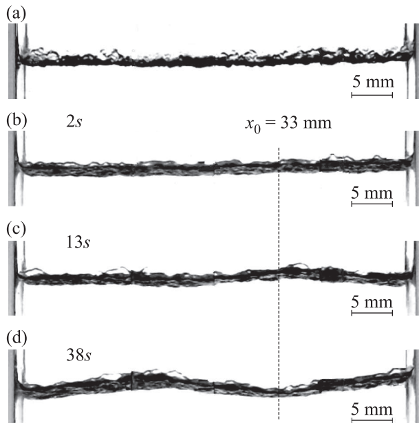
Рис. 2. Фотографии поверхности при различных режимах ультразвукового облучения. (a) – Немодулированный ультразвук. (b)–(d) – Последовательные стадии развития колебаний при частотной модуляции ультразвука. Указано время от начала возбуждения. Штриховой линией обозначено вертикальное сечение для нахождения функции смещения поверхности во времени
